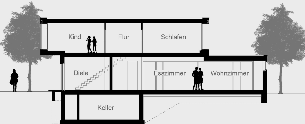
Schnitt B-B
