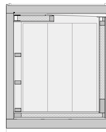
Querschnitt _ 1/50 _ Transportposition
