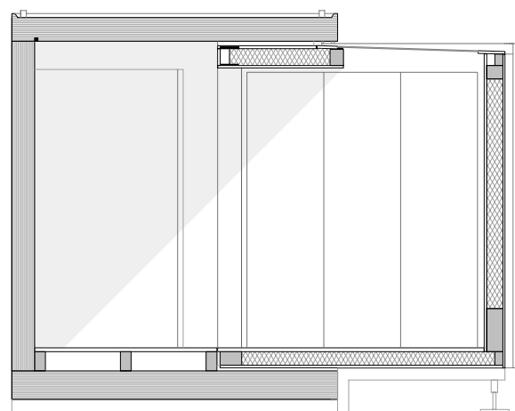
Querschnitt _ 1/50 _ Ausstellungsposition
