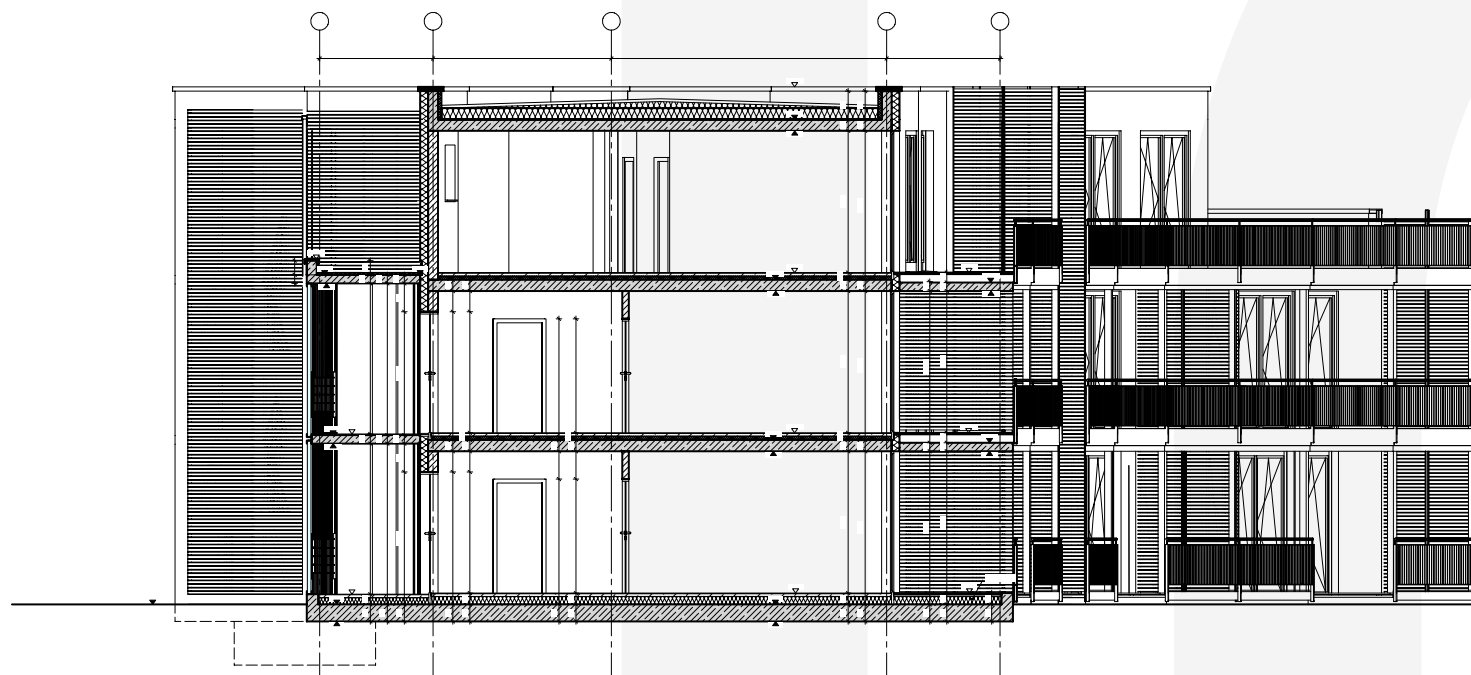
Querschnitt Wohnungen
