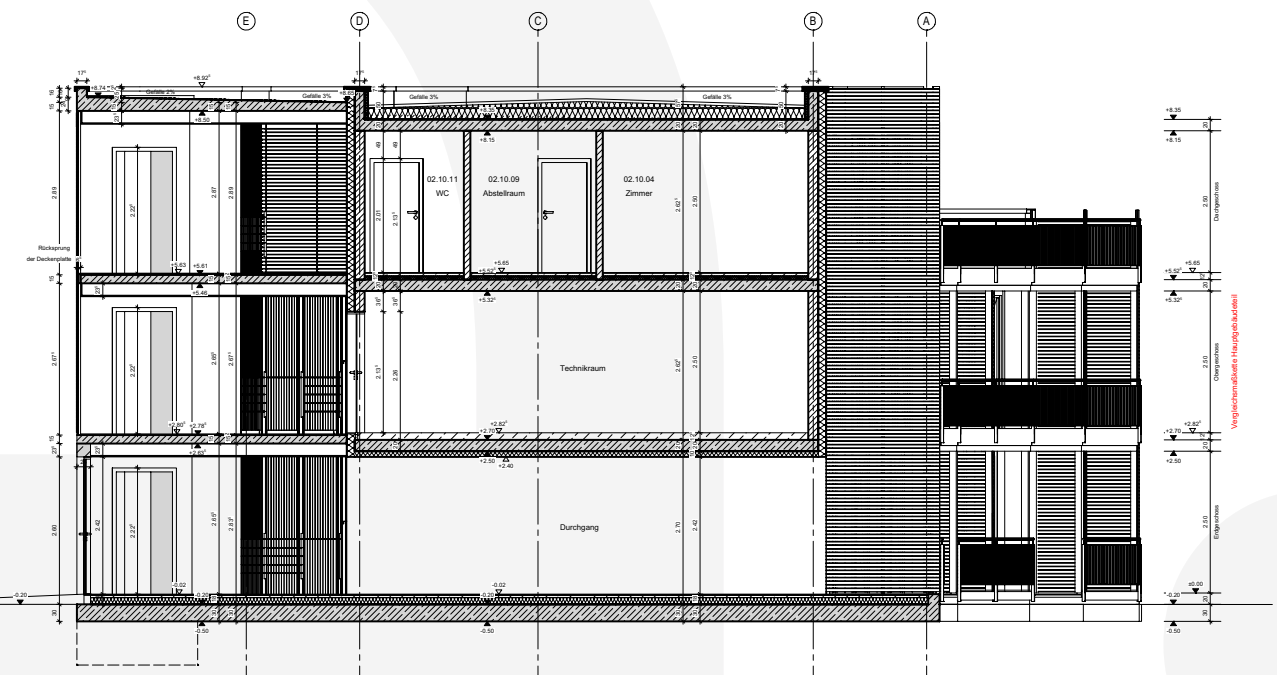
Querschnitt Erschließung
