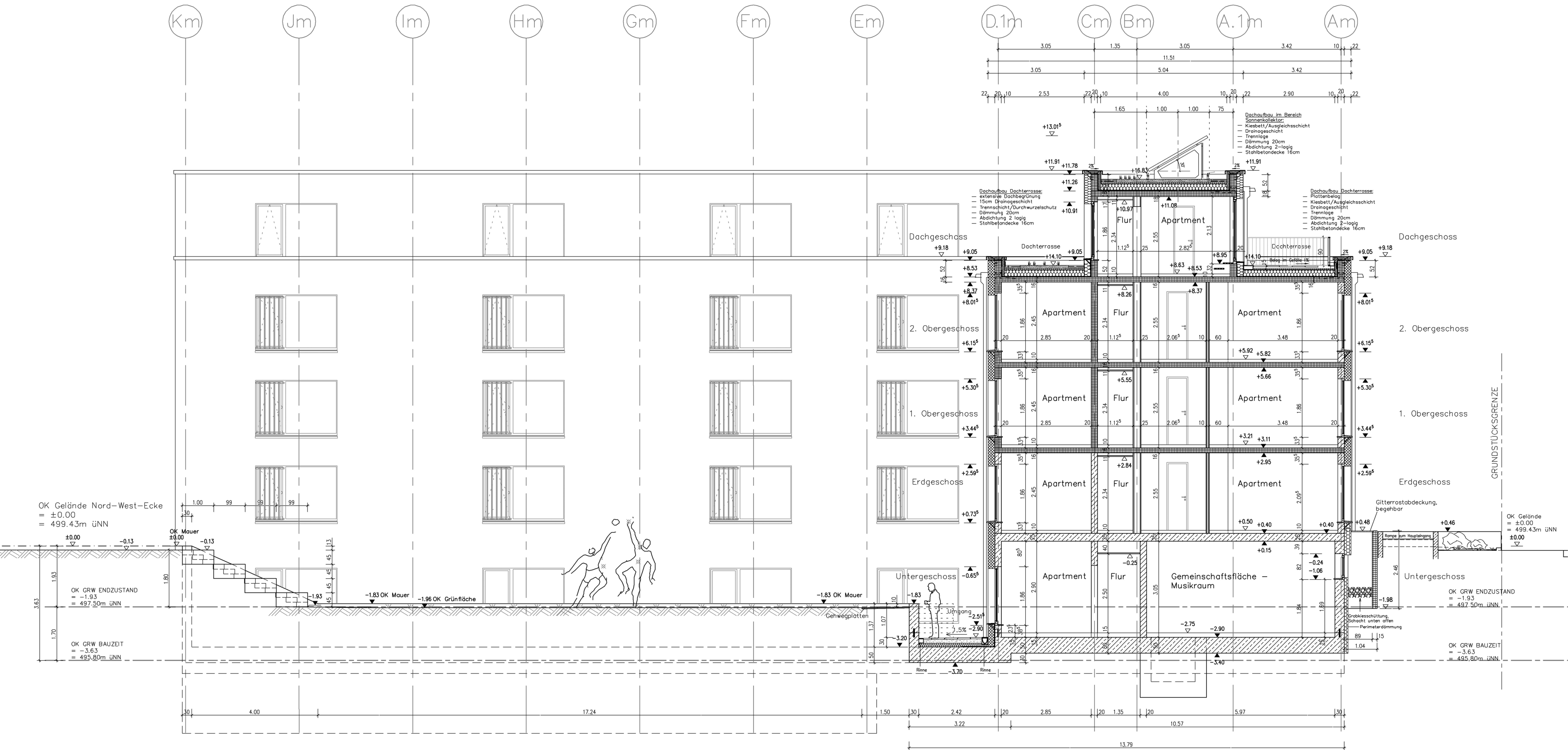
SCHNITT D - D
