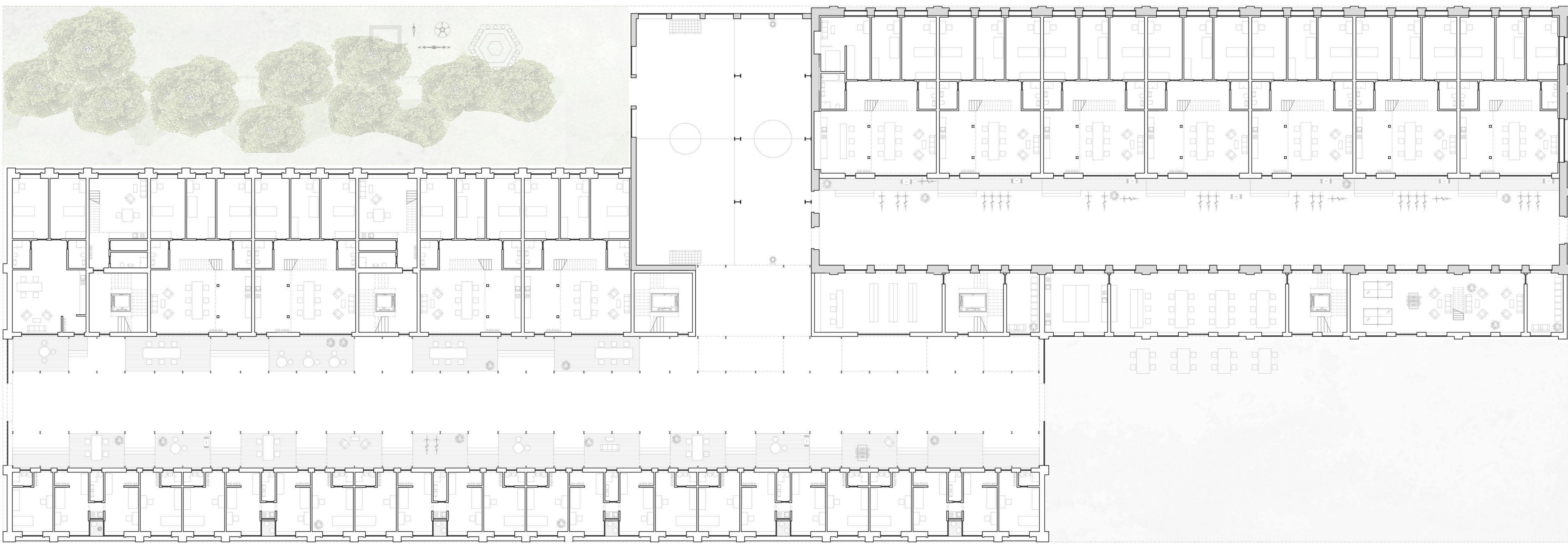
GRUNDRISS EG M 1: 200
