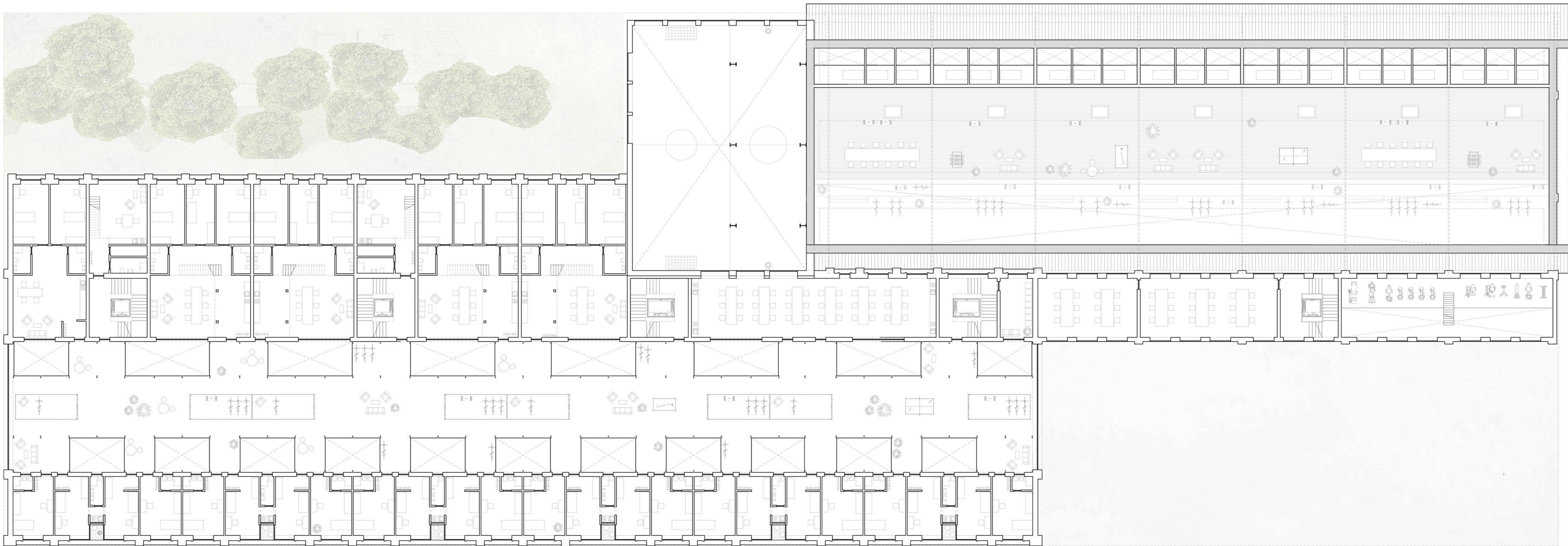
GRUNDRISS 2. OG M 1:200
