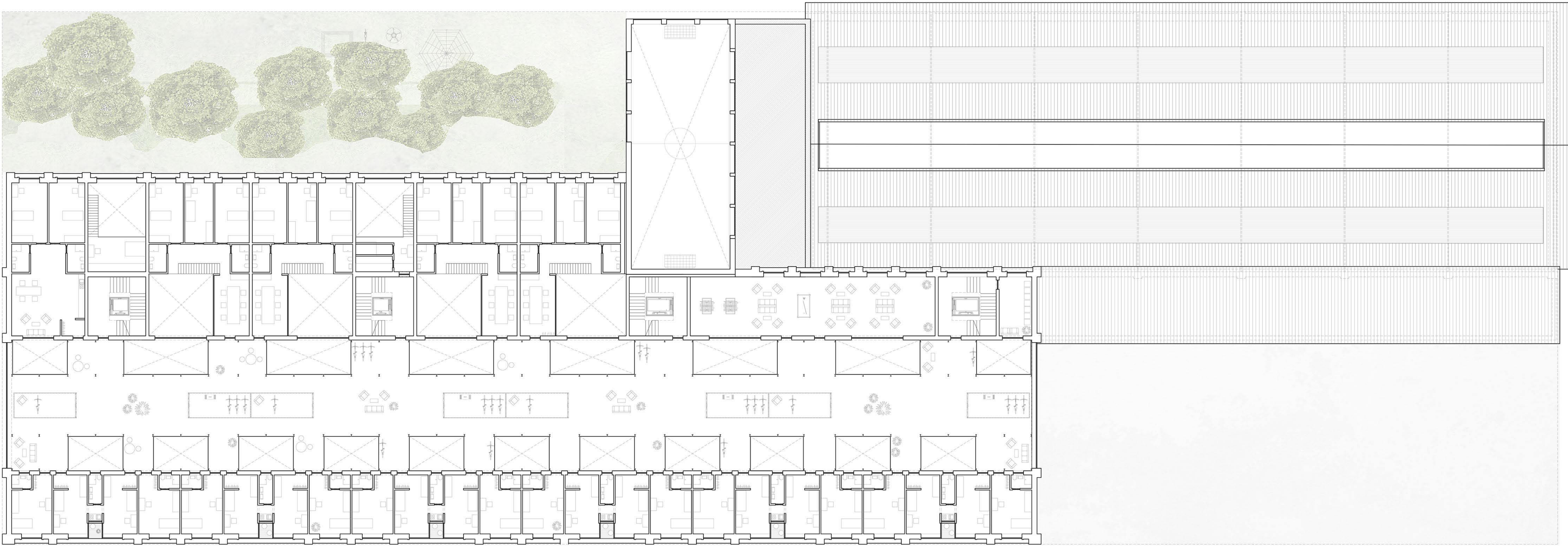
Grundriss 3. OG M 1:200
