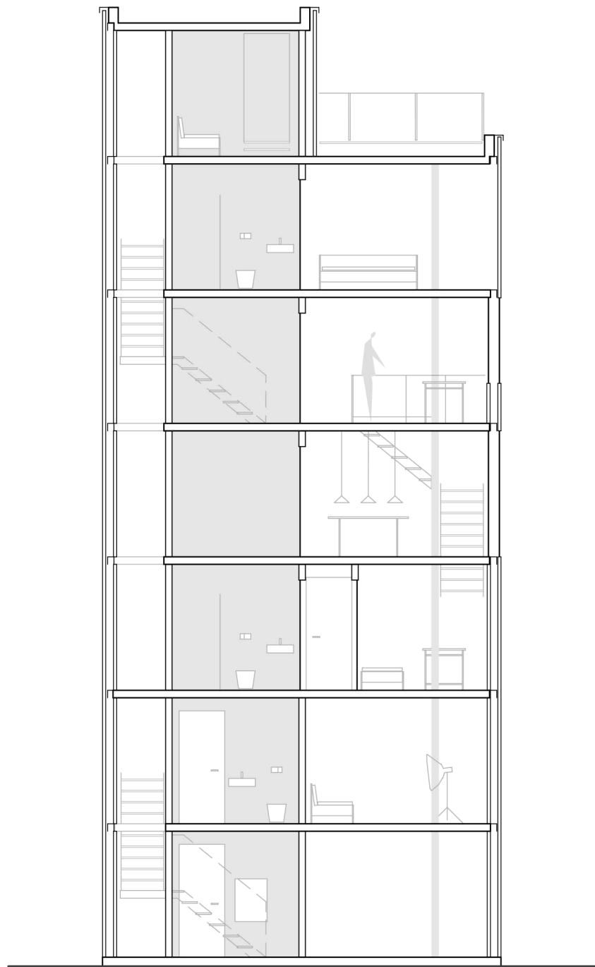
Längsschnitt 1 zu 100
