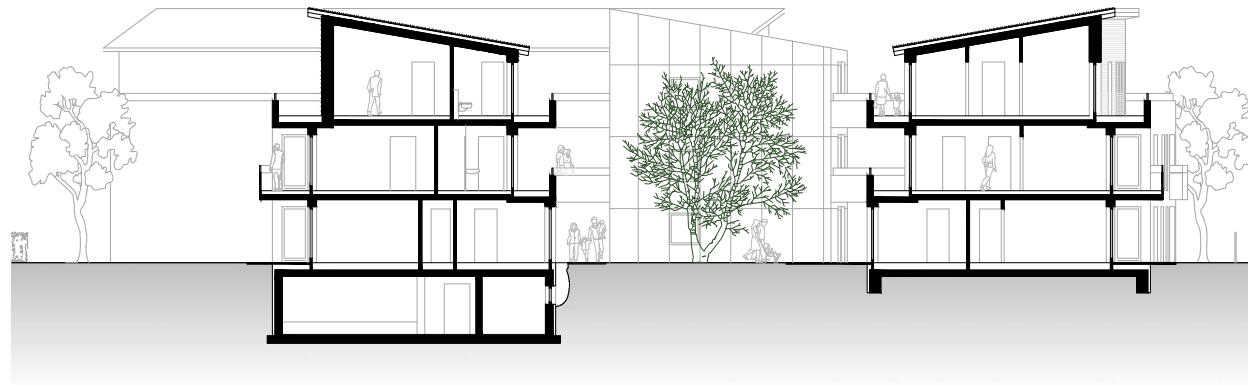
GEBÄUDESCHNITT
