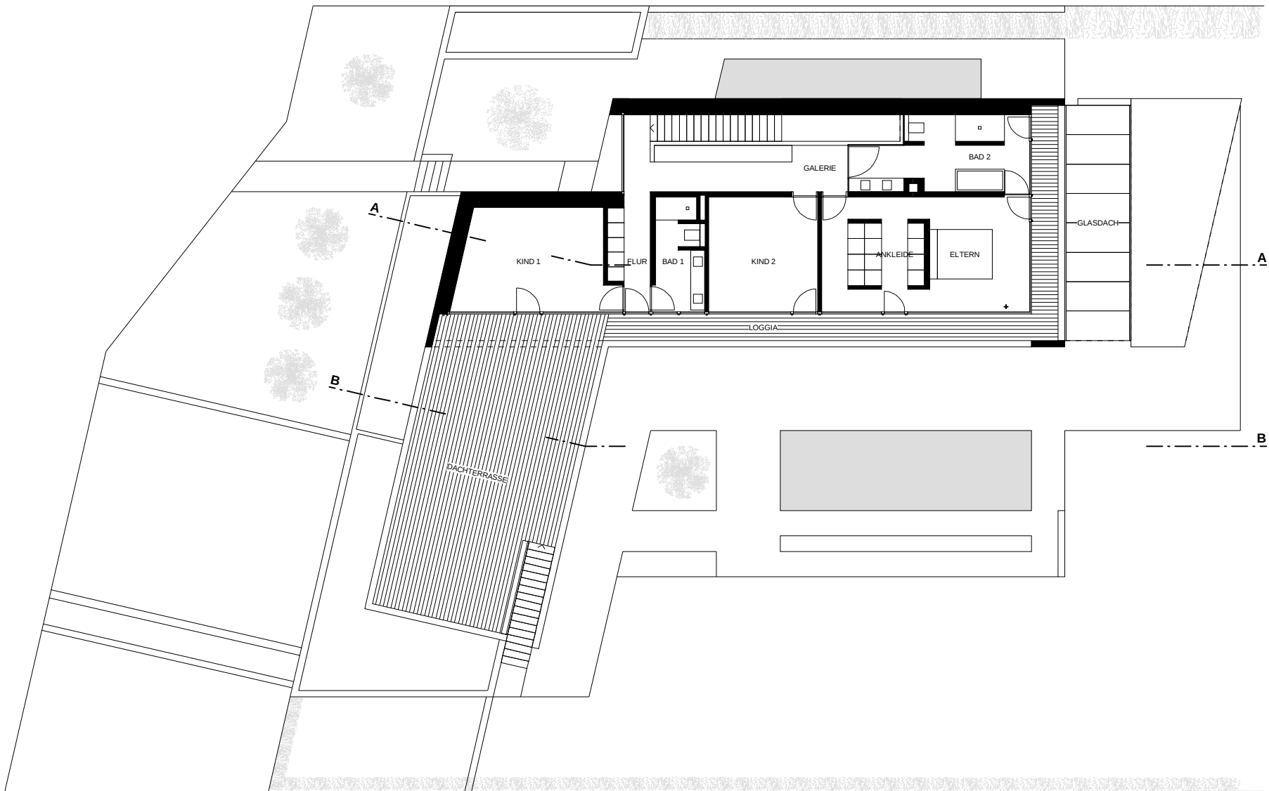
GRUNDRISS OG
