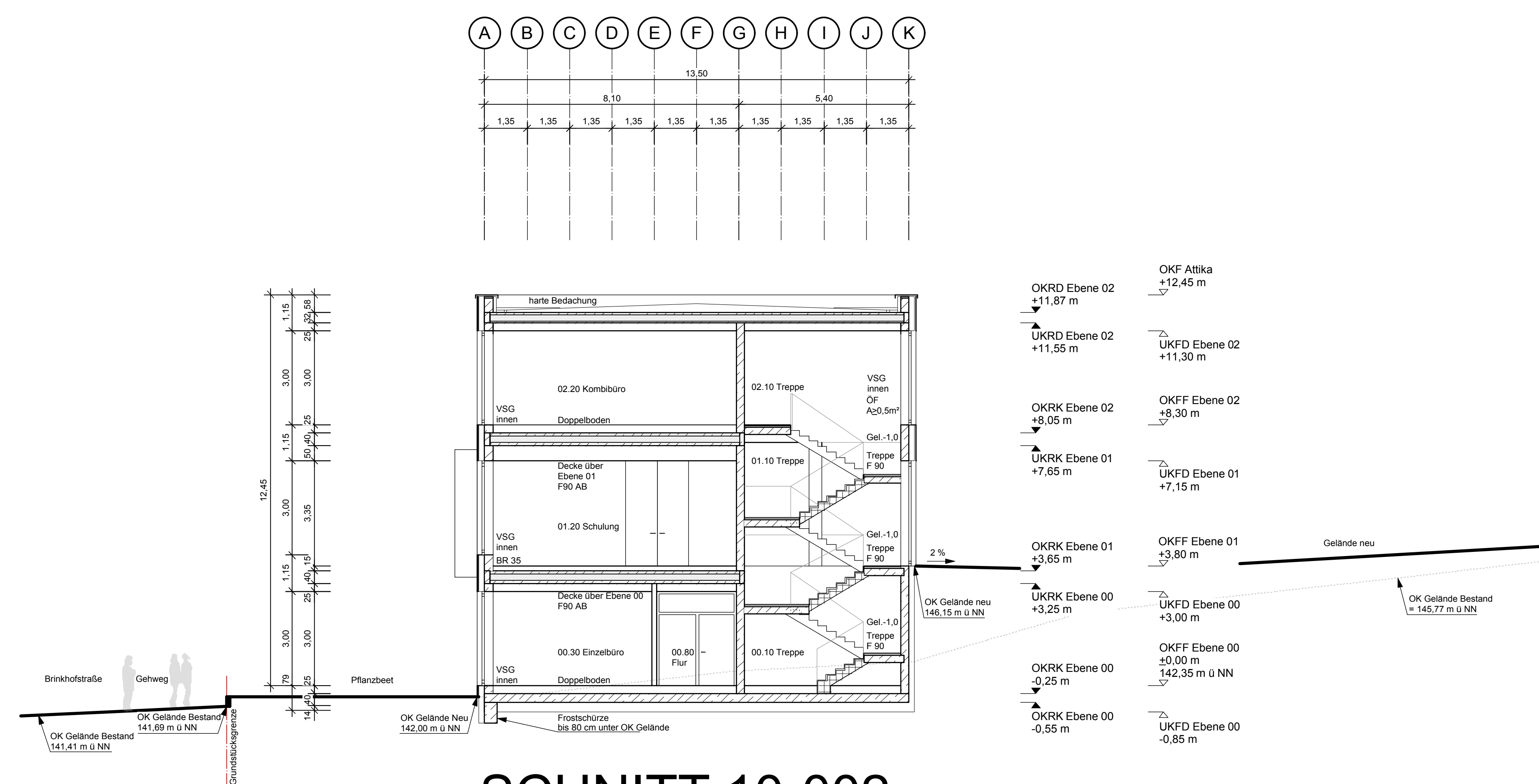
SCHNITT 10-002
