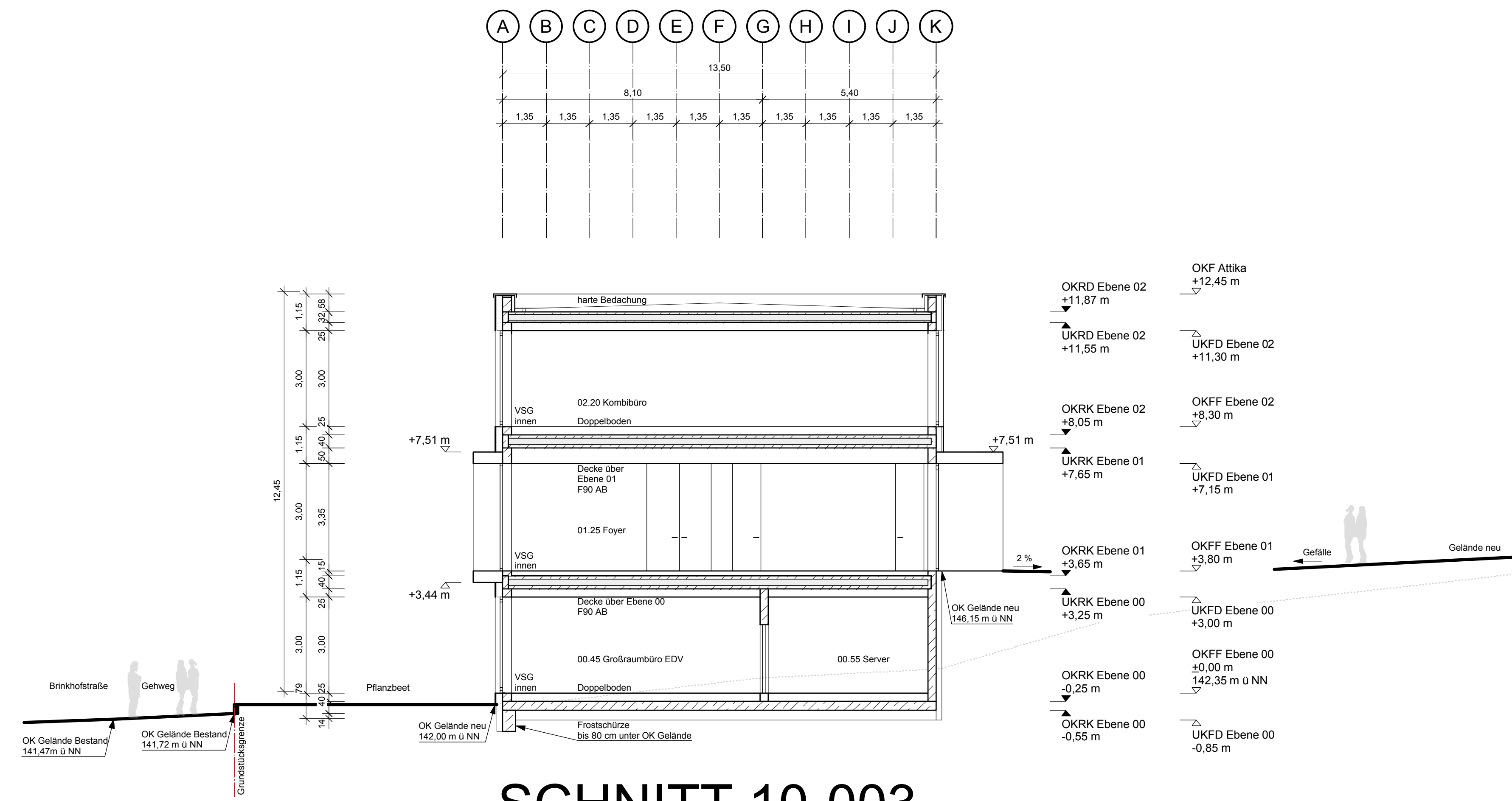
SCHNITT 10-003
