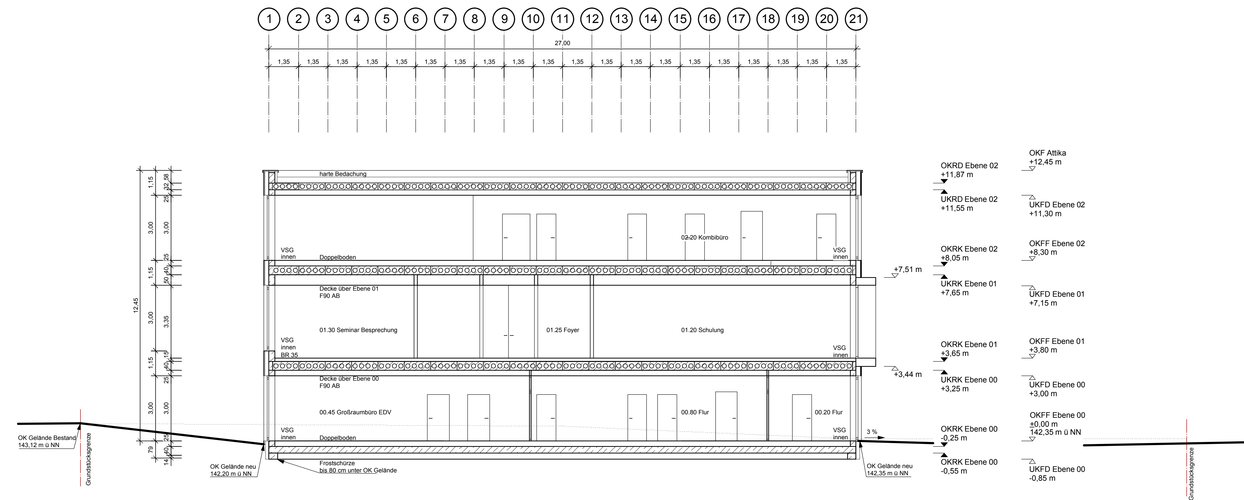
SCHNITT 10-001
