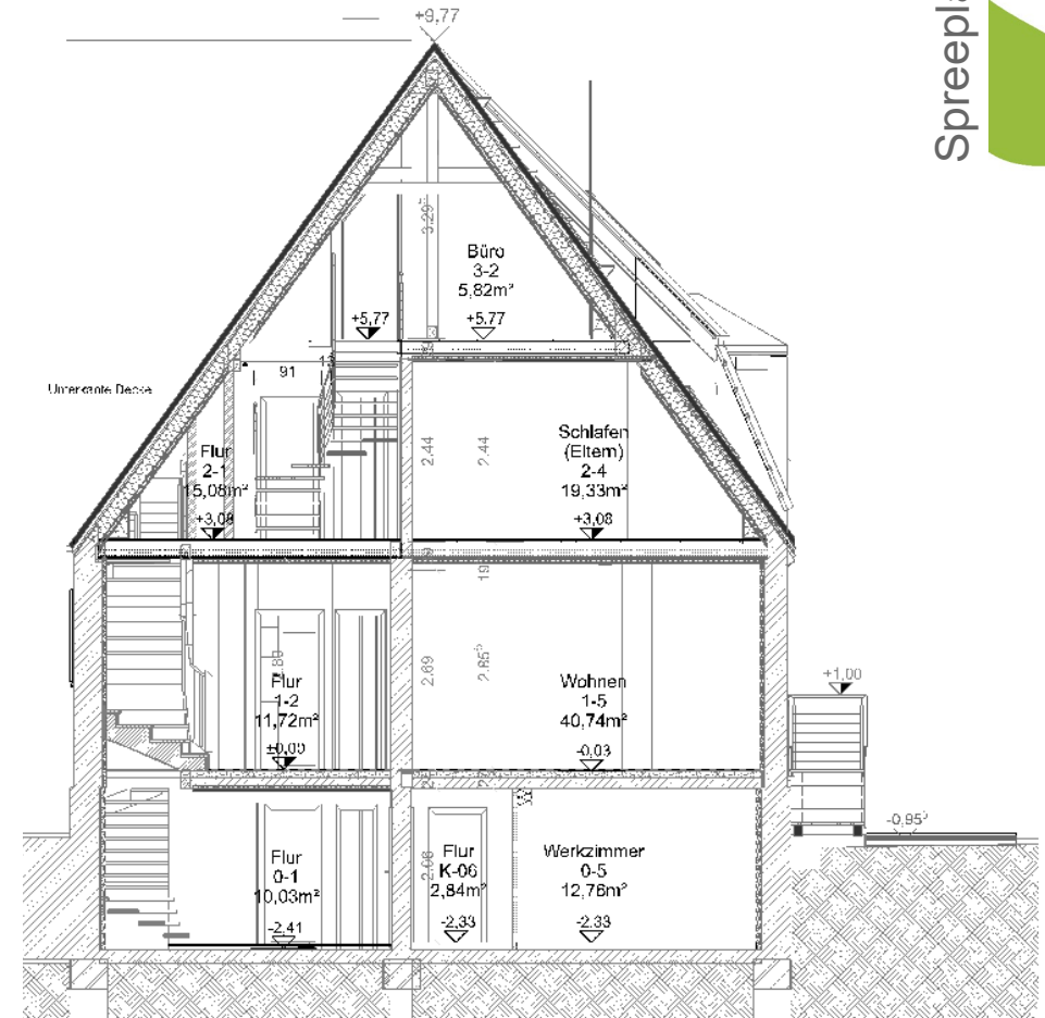
Schnitt B-B
