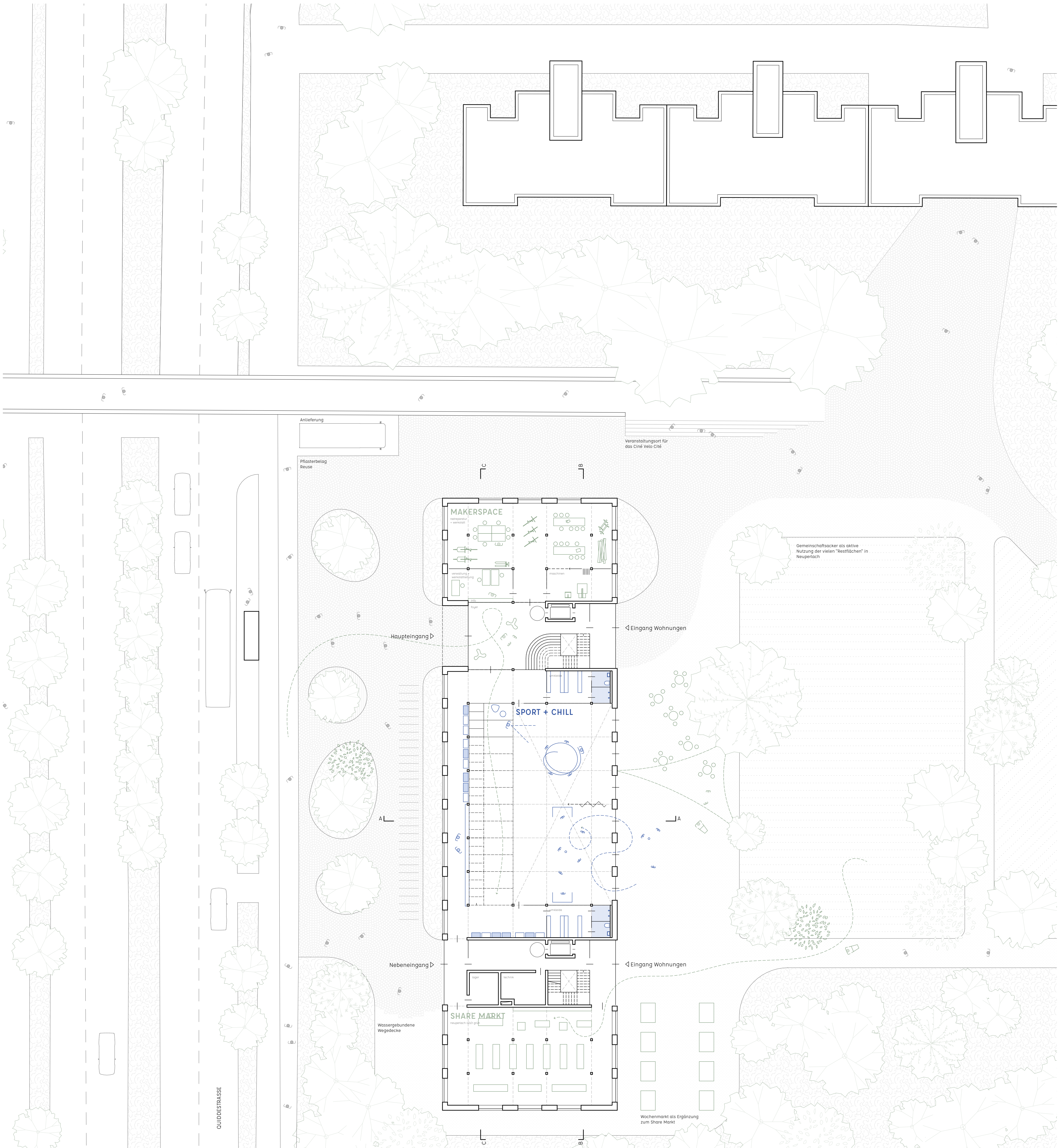
Grundriss EG mit Umgriff M 1:200
