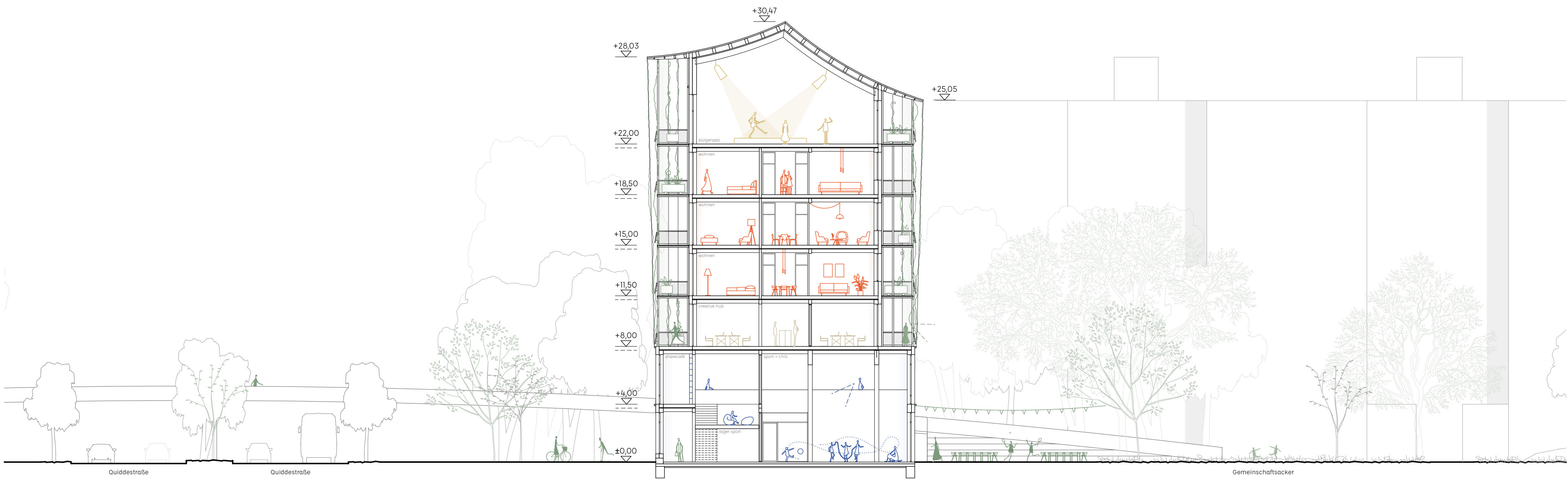
Schnitt A M 1:200
