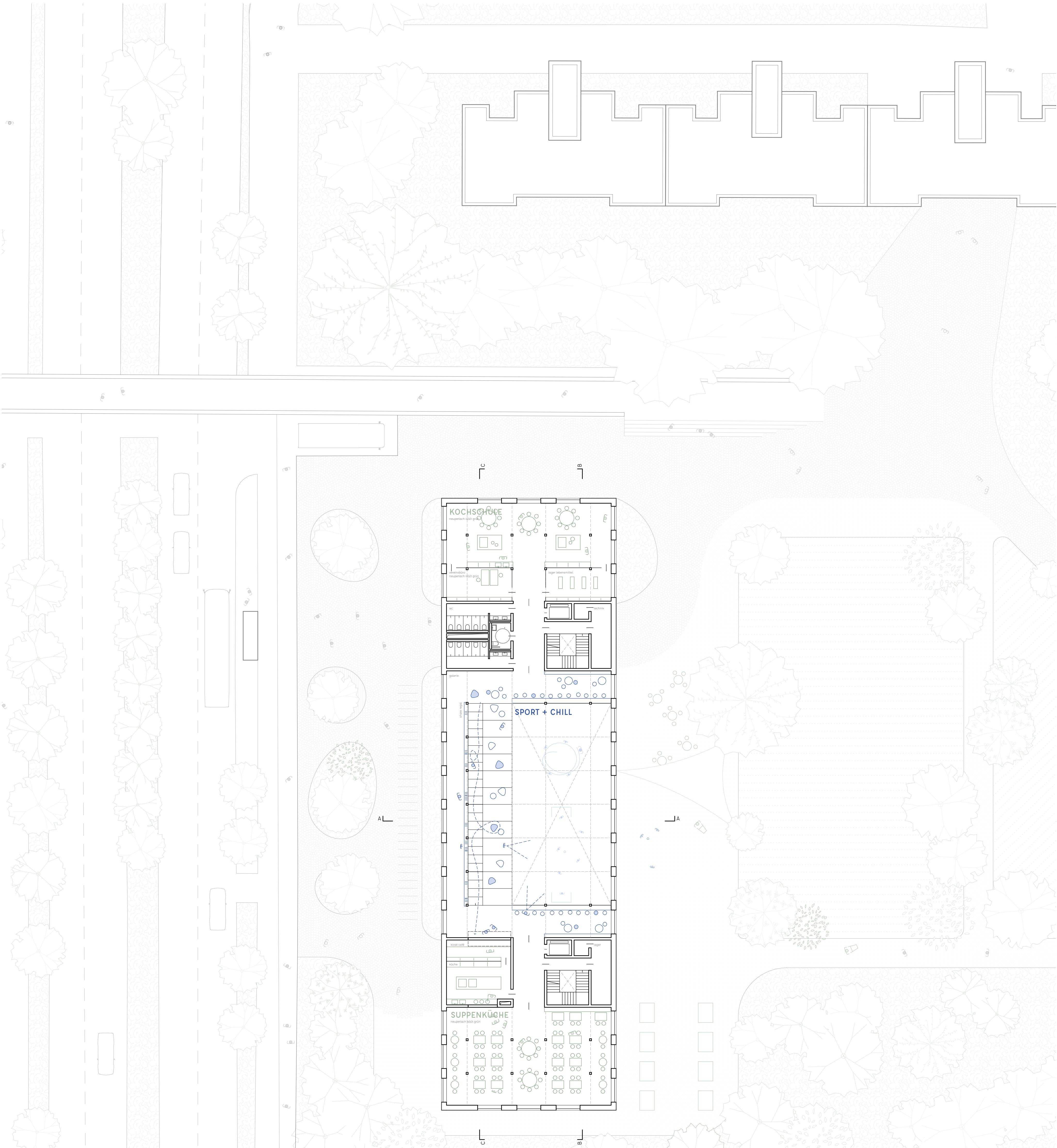
Grundriss OG 01 mit Umgriff M 1:200
