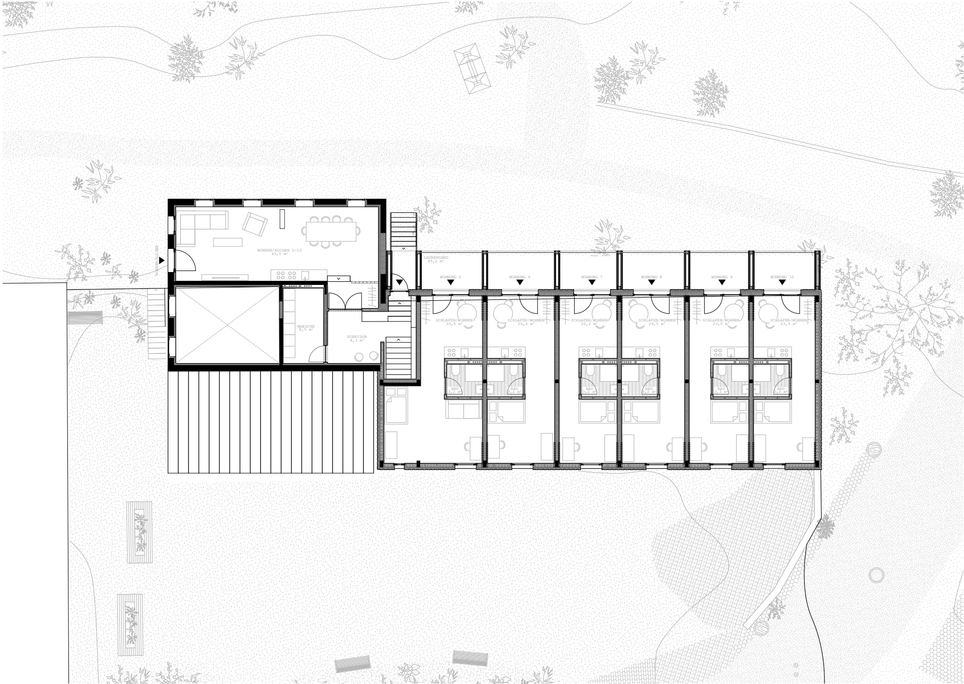
Wagenhalle Ebene 2
