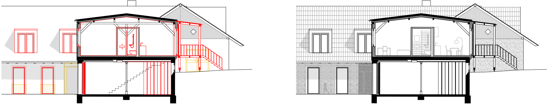
Querschnitt Wagenhalle
