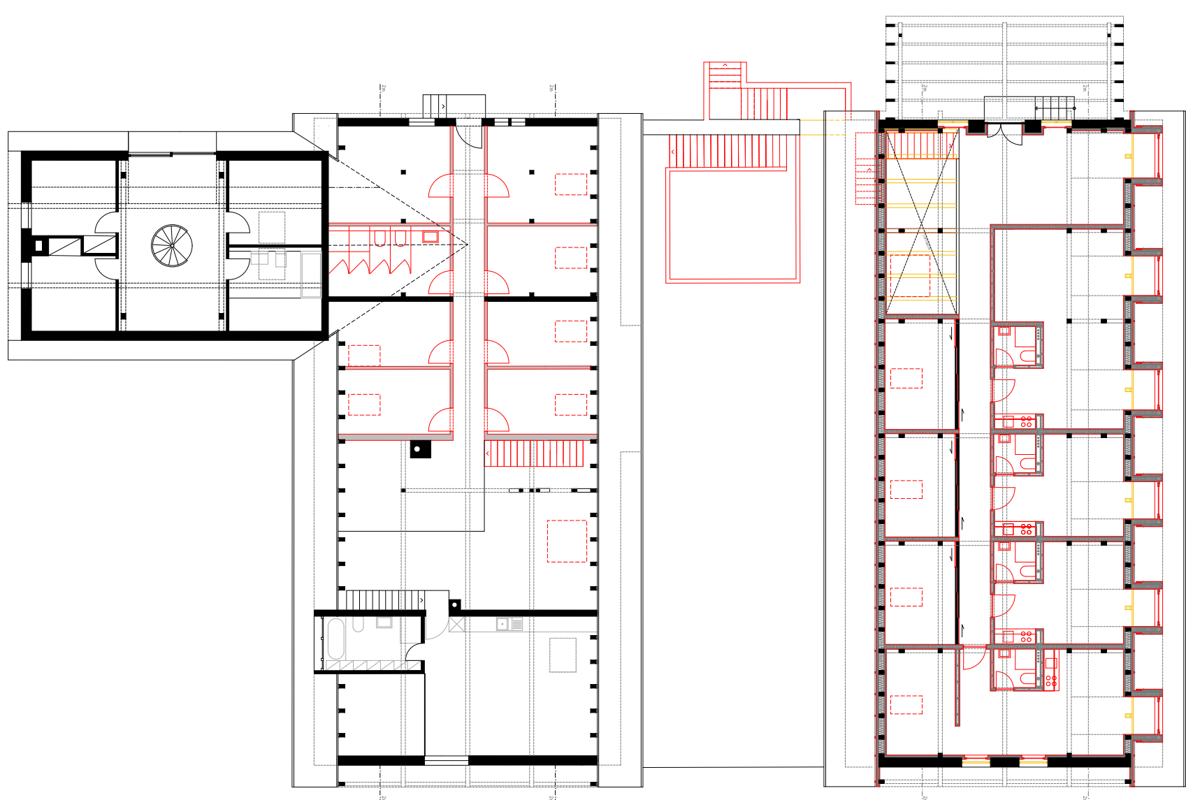
Käsererei Ebene 2 Neubau/Abriss
