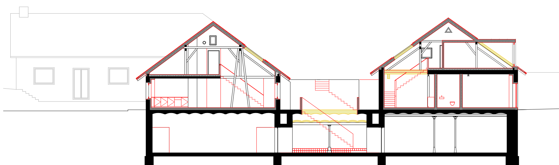
Käsererei Querschnitt Neubau/Abriss
