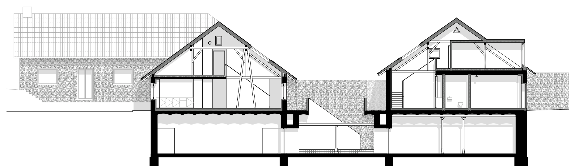
Käsererei Querschnitt
