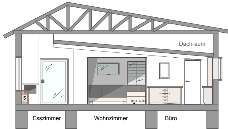
Schnitt AA'
