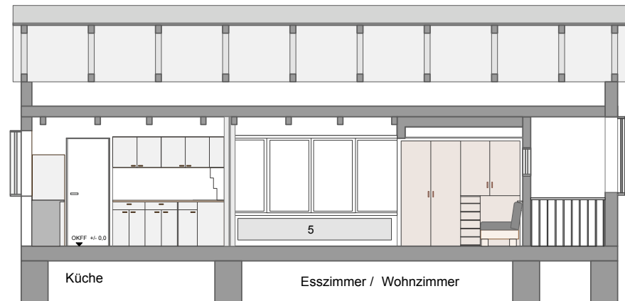
Schnitt DD'
