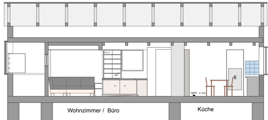
Schnitt CC'
