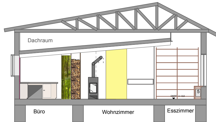
Schnitt BB'
