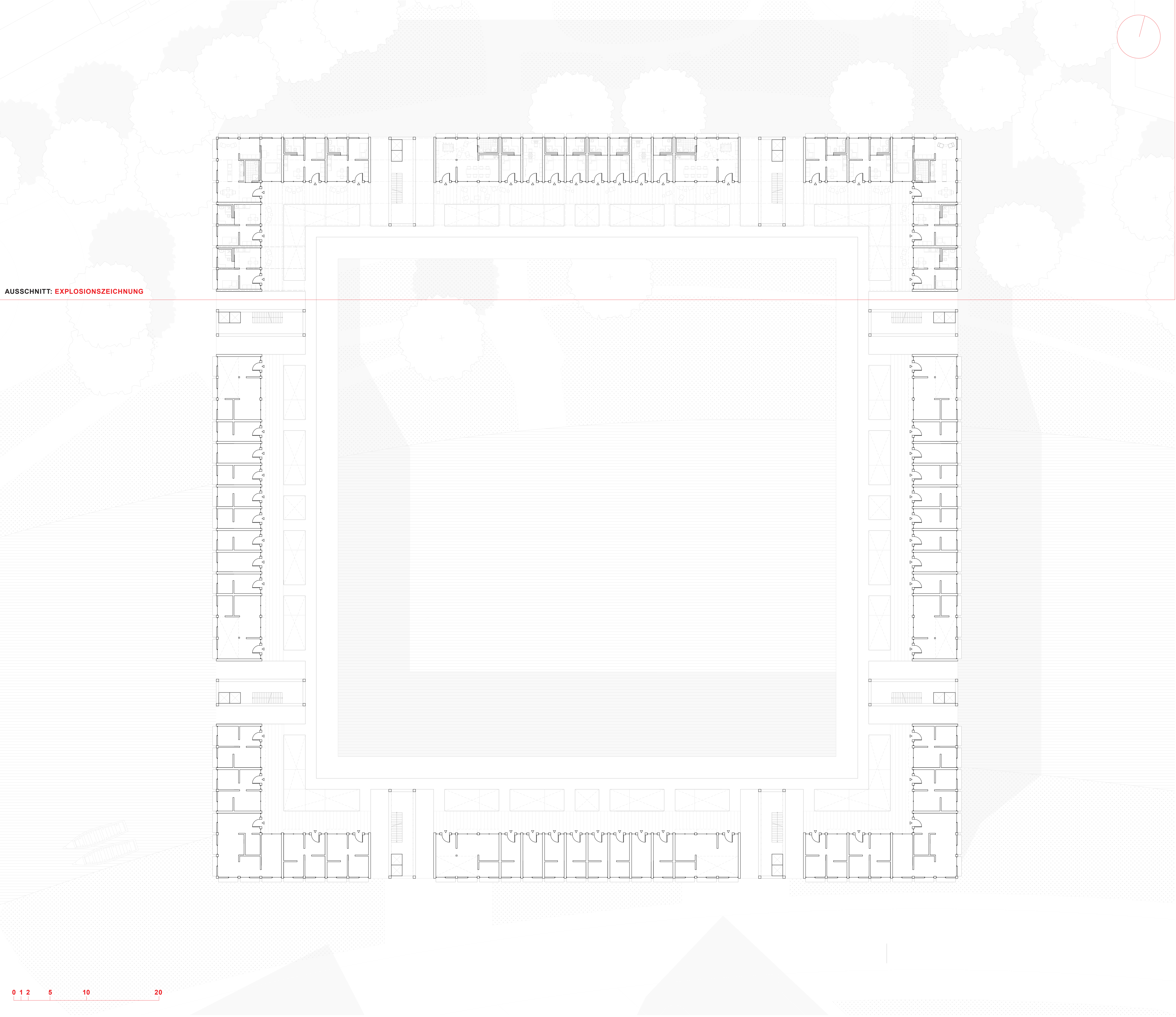
GRUNDRISSE OG 2: 1 : 200
