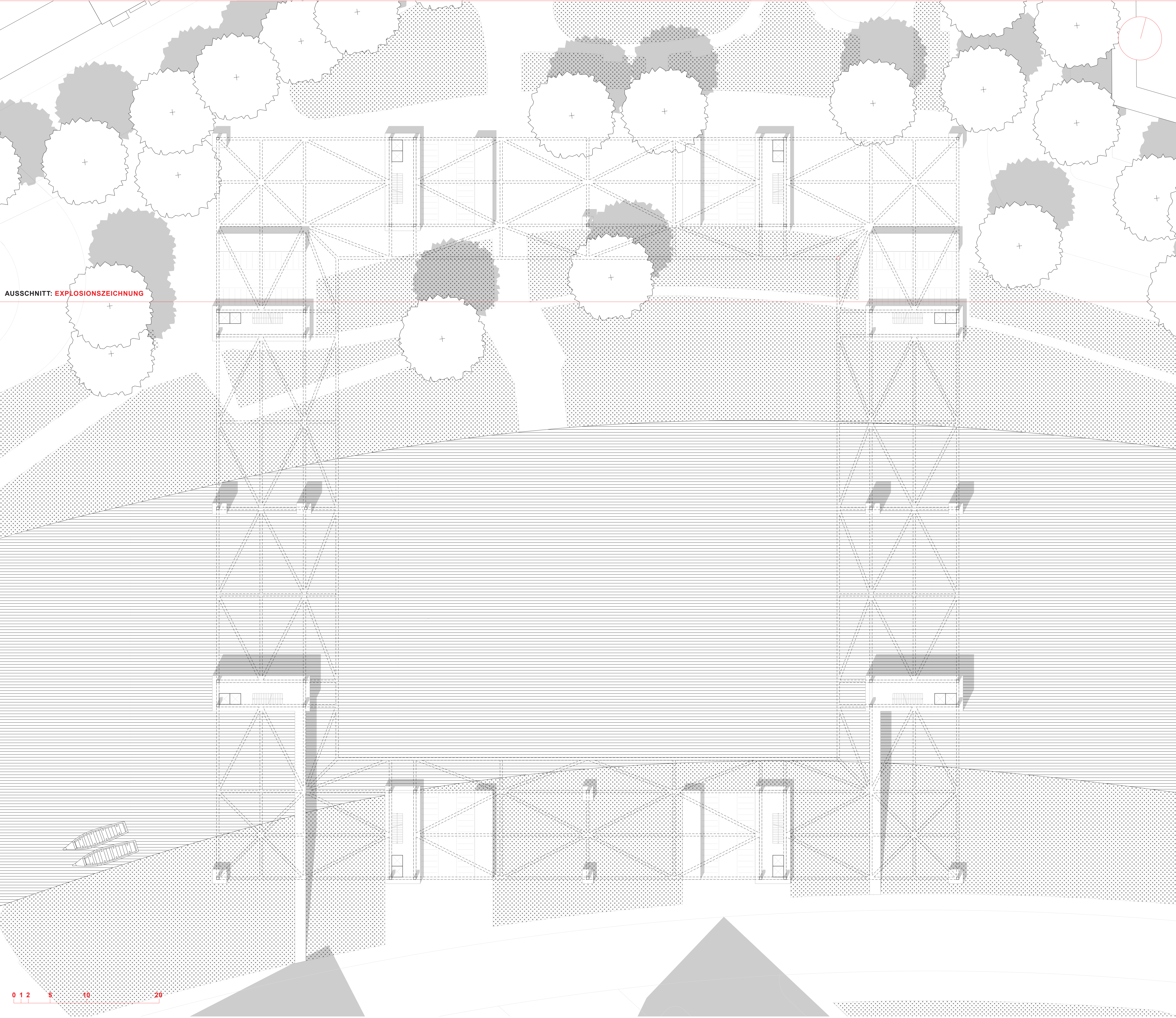
GRUNDRISS EG 1: 1 : 200
