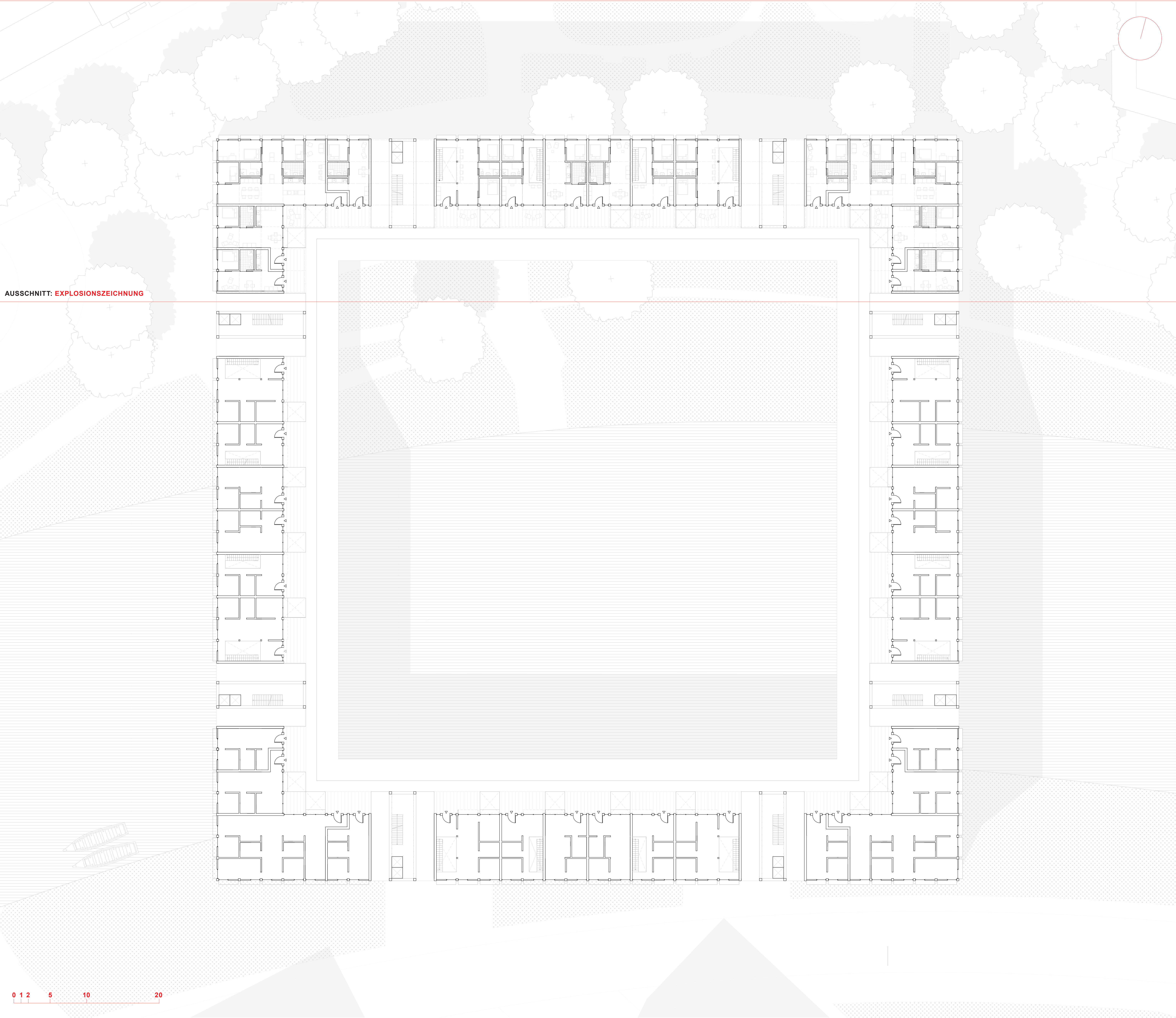
GRUNDRIS OG 1: 1 : 200
