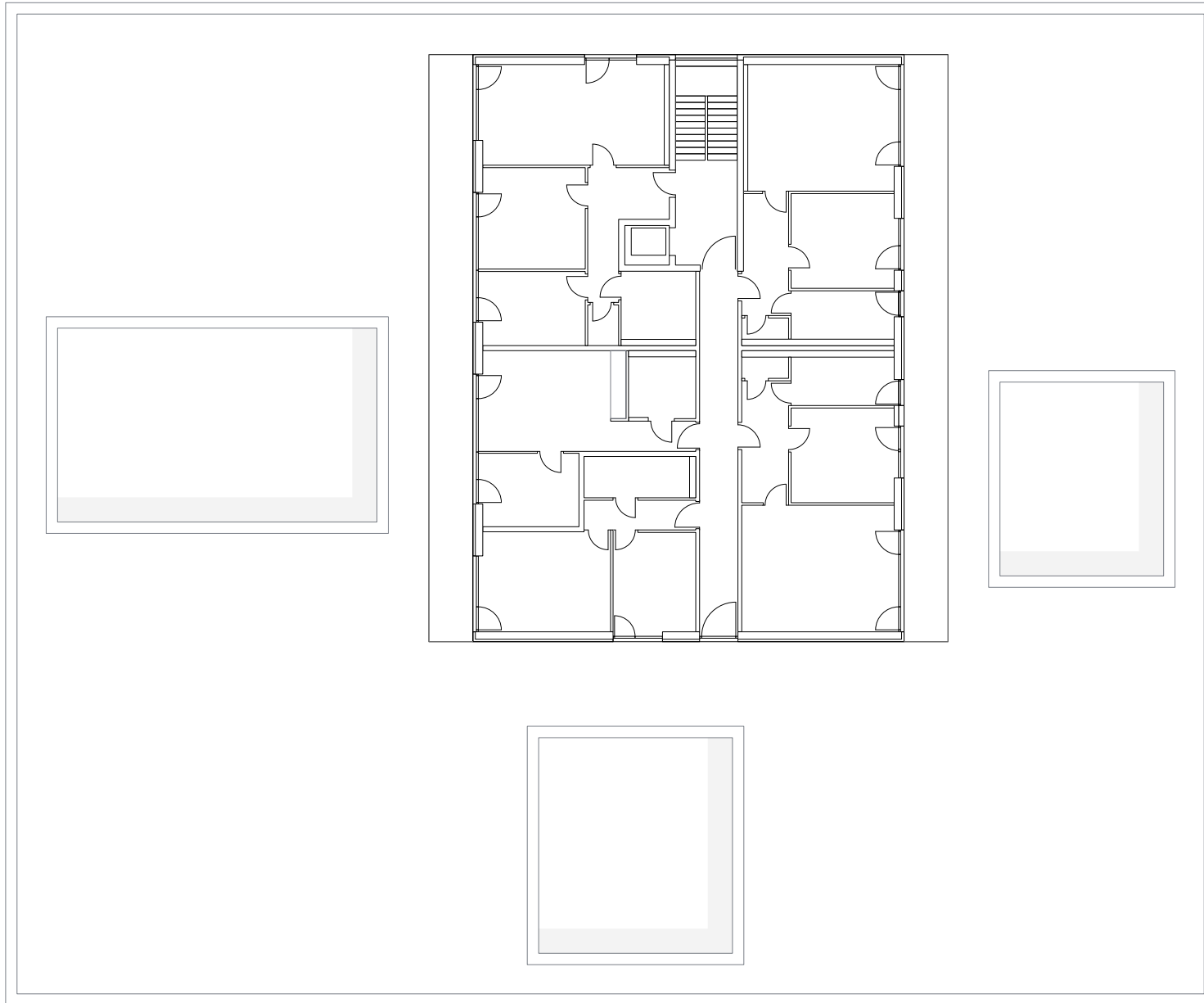
Grundriss OG
