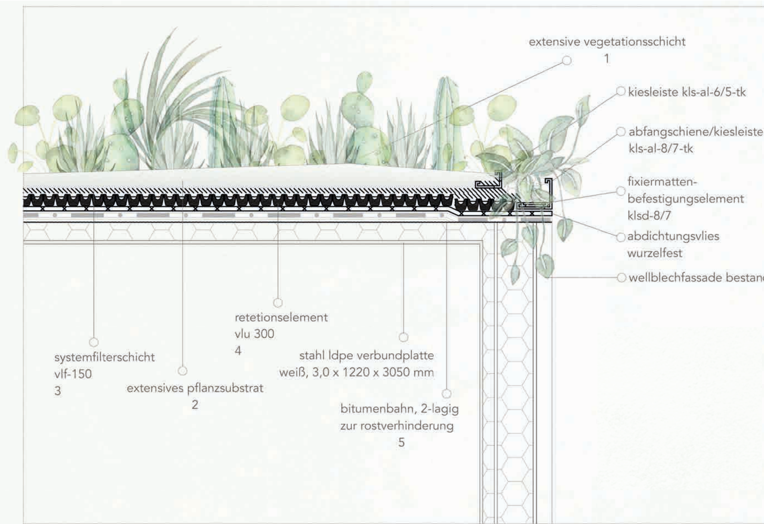
schnitt
