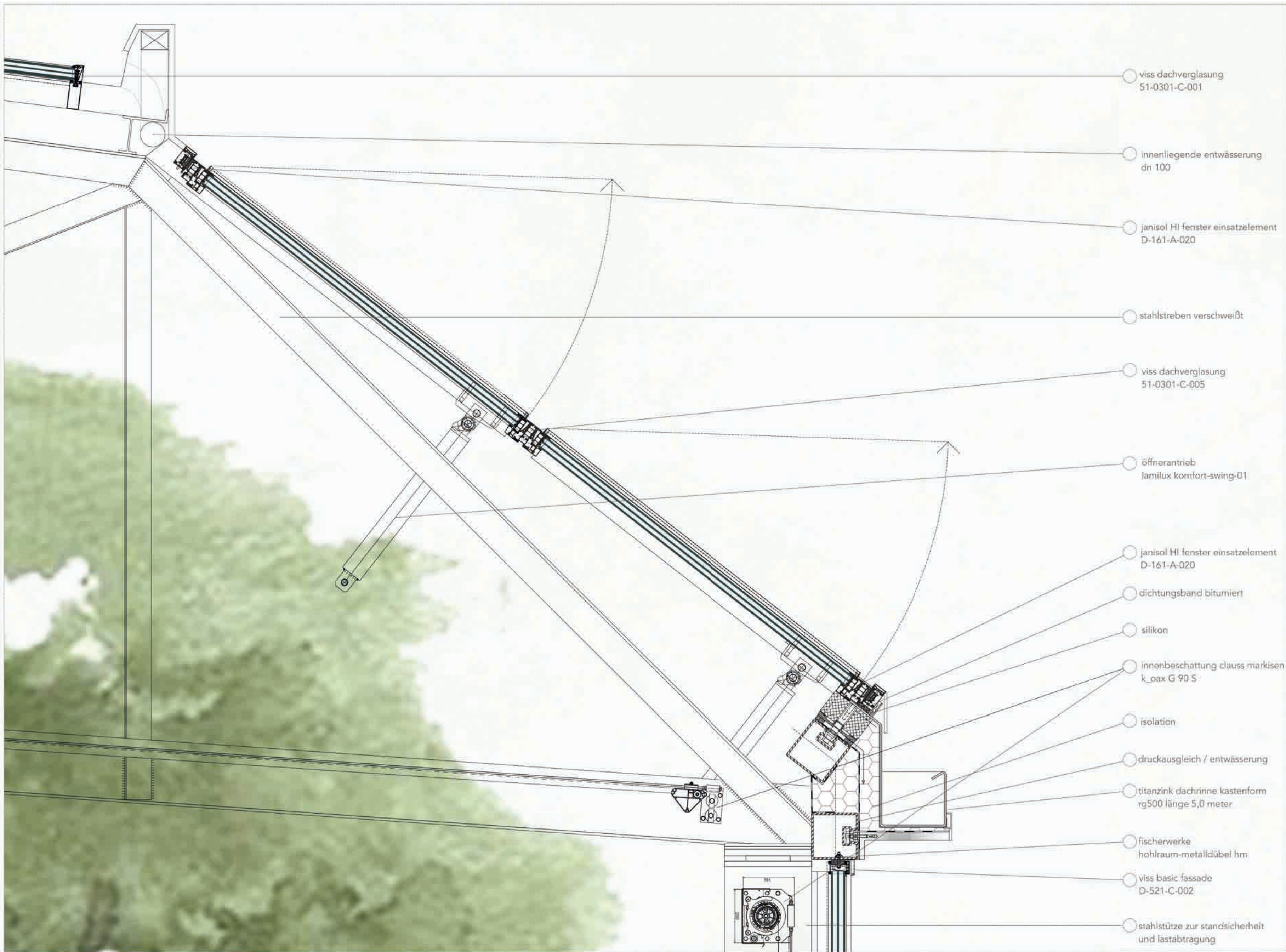
schnitt
