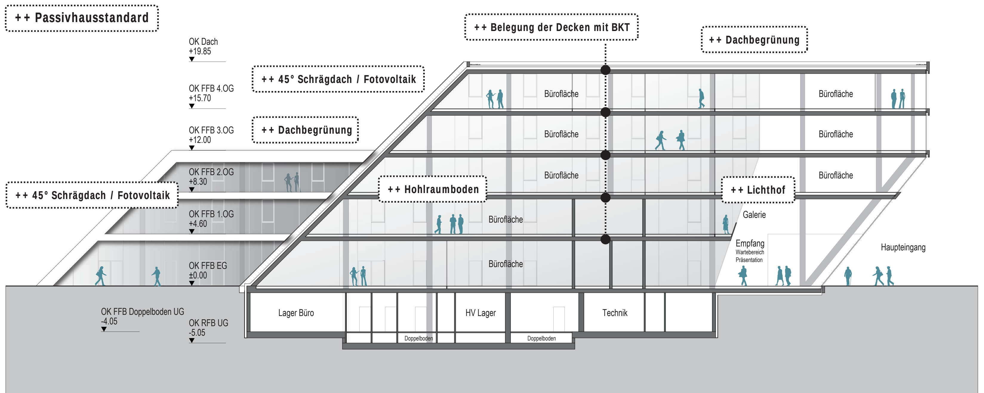
Schnitt AA . M 1:200
