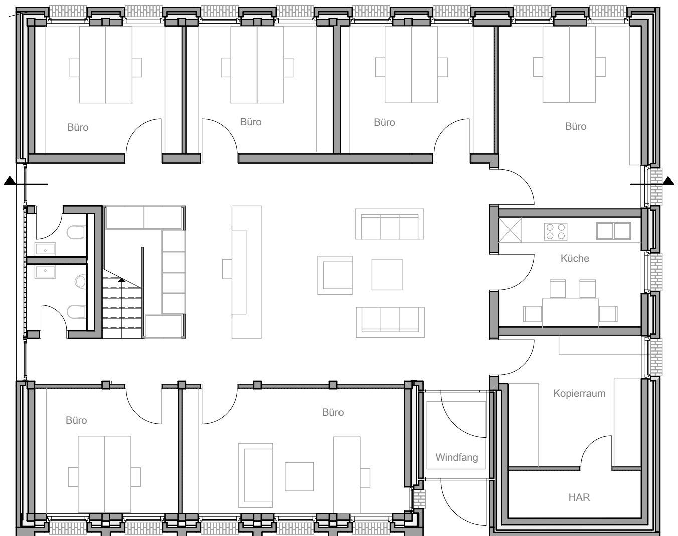
Grundriss EG
