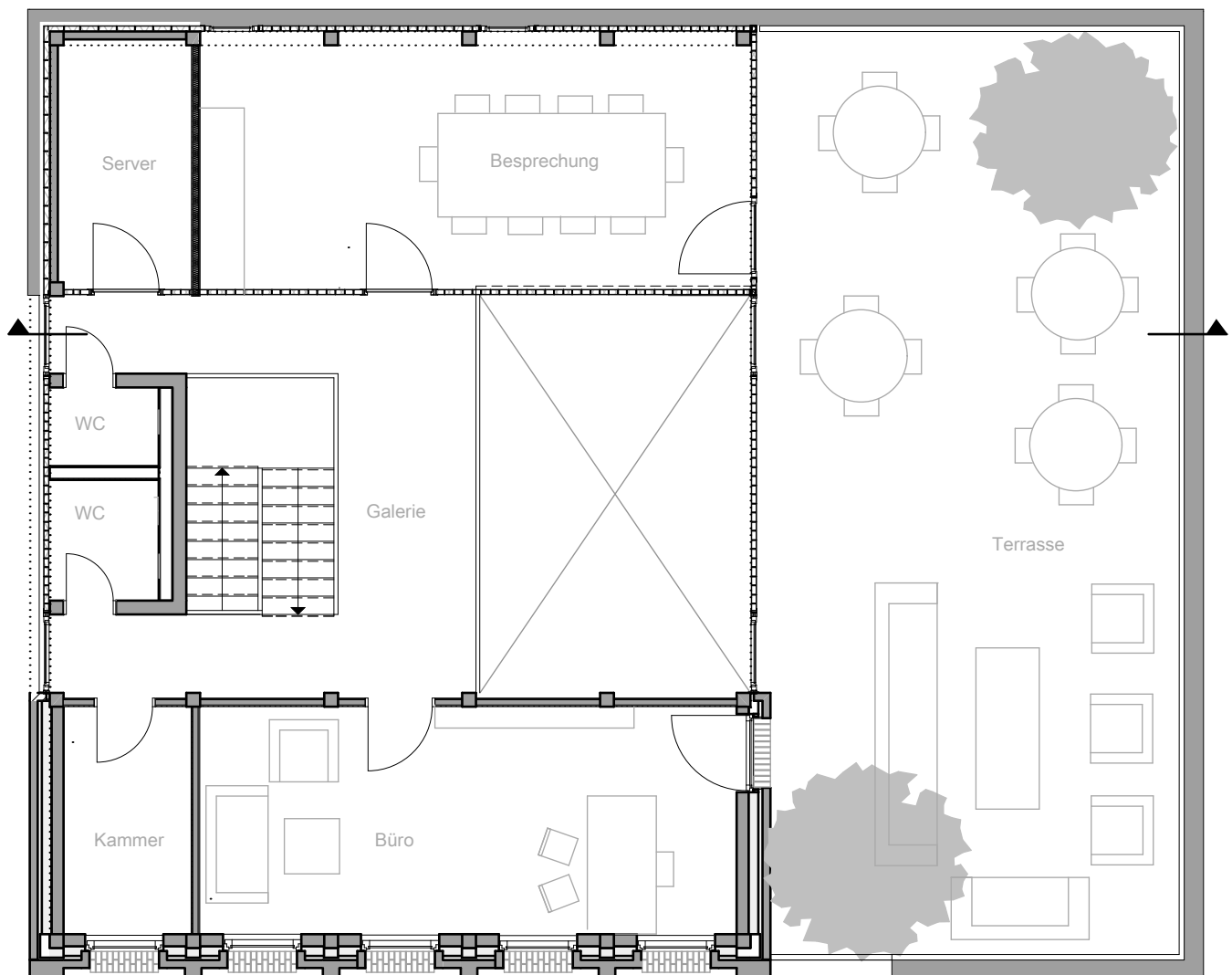
Grundriss OG
