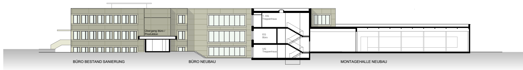
SCHNITT A-A
