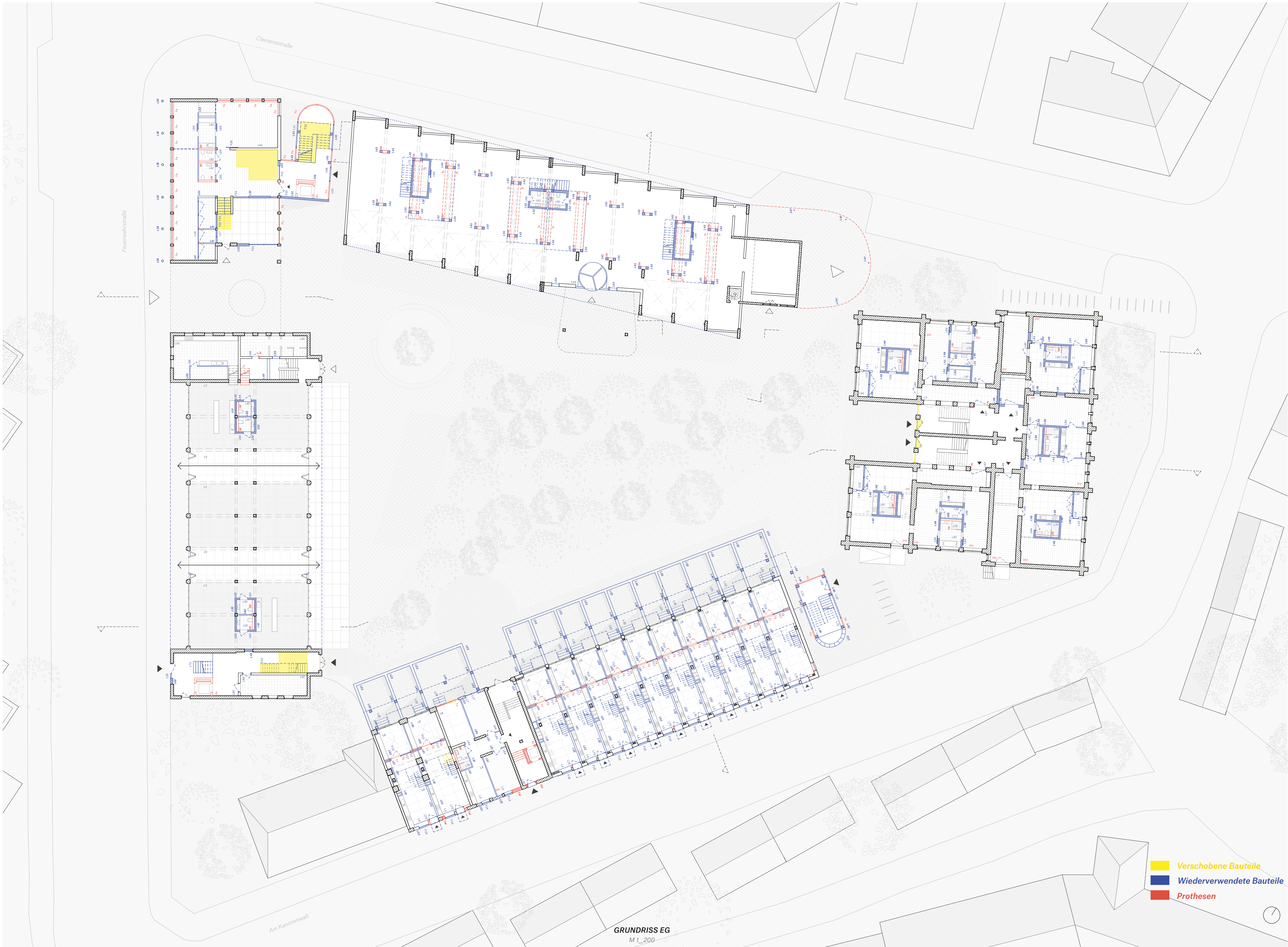
PHASE 3: NEUBAU ERSETZT DURCH BAUTEILE EG M 1_750
