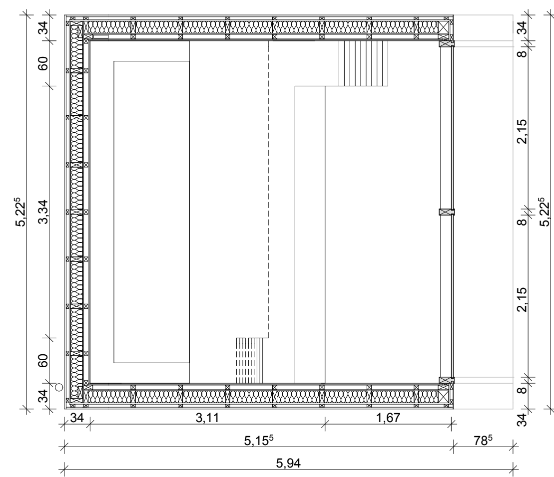
GRUNDRISS 1. OG M 1:50
