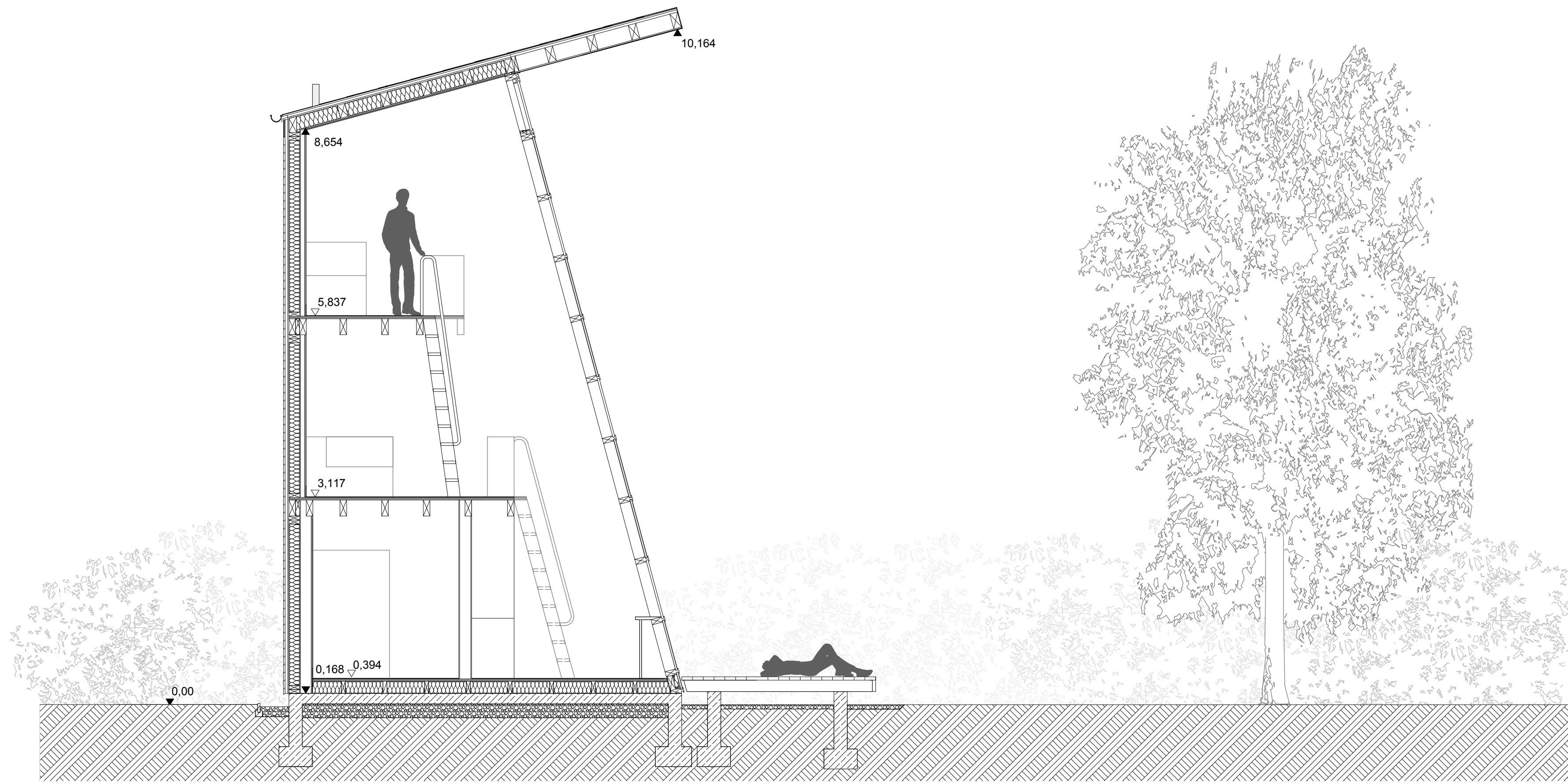
SCHNITT M 1:50
