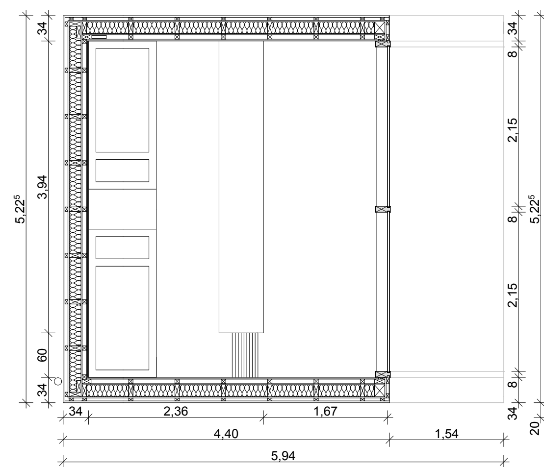
GRUNDRISS 2. OG M 1:50
