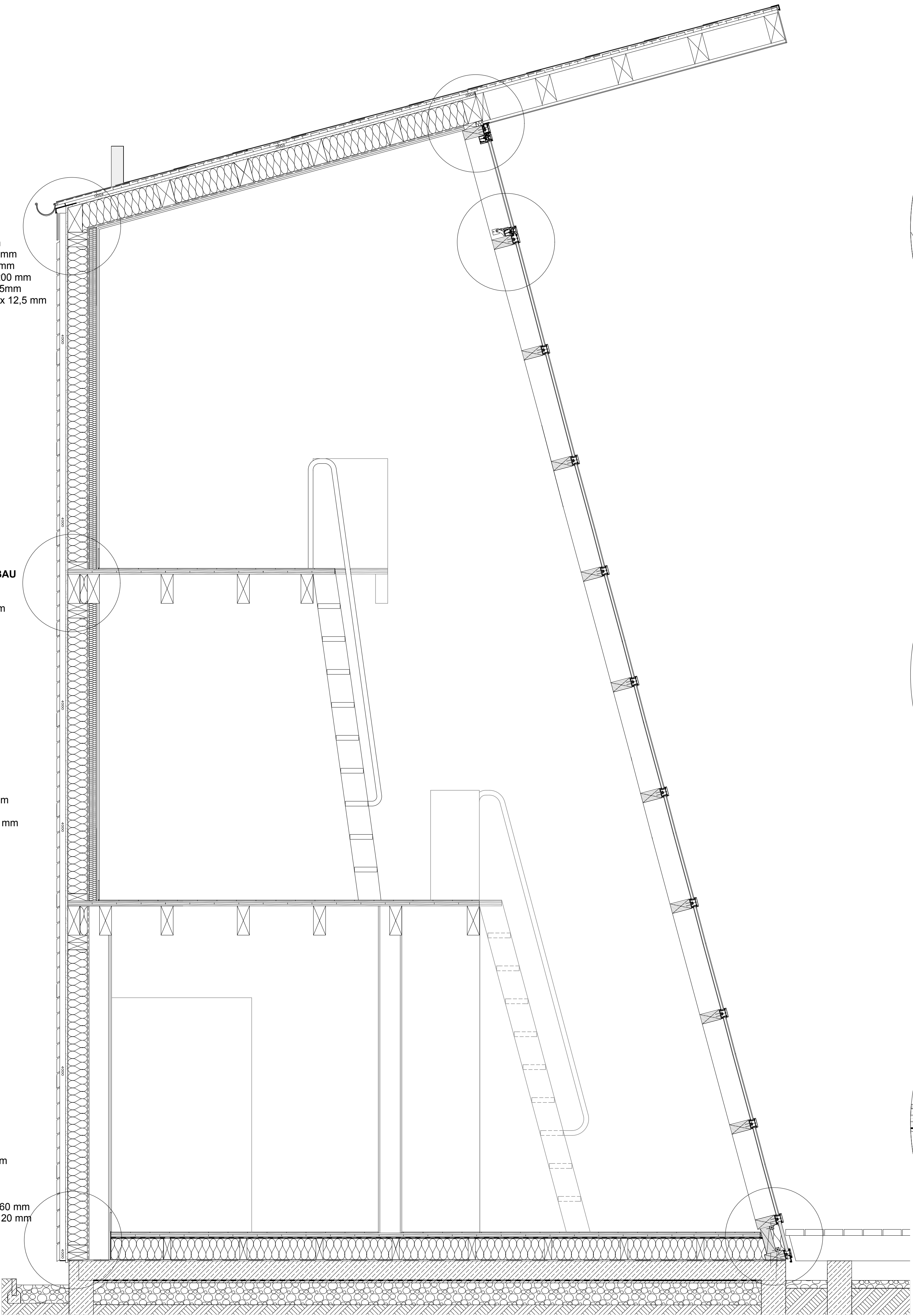
FASSADENSCHNITT 1: 20
