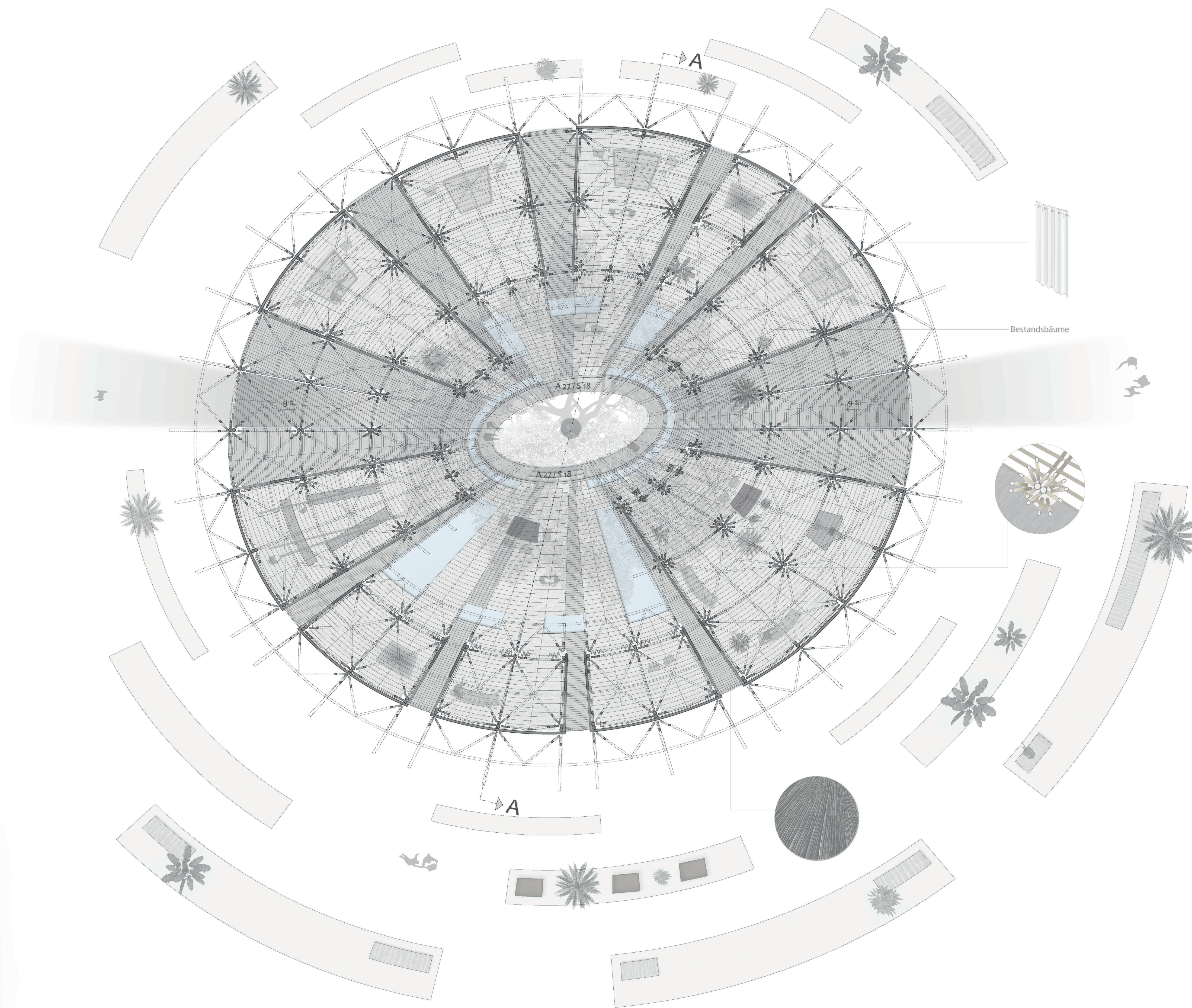
Grundriss 1:100
