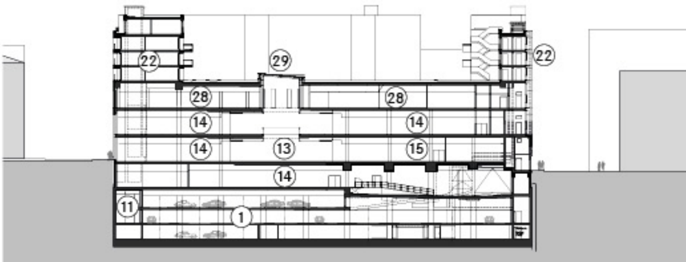
Schnitt Q6
