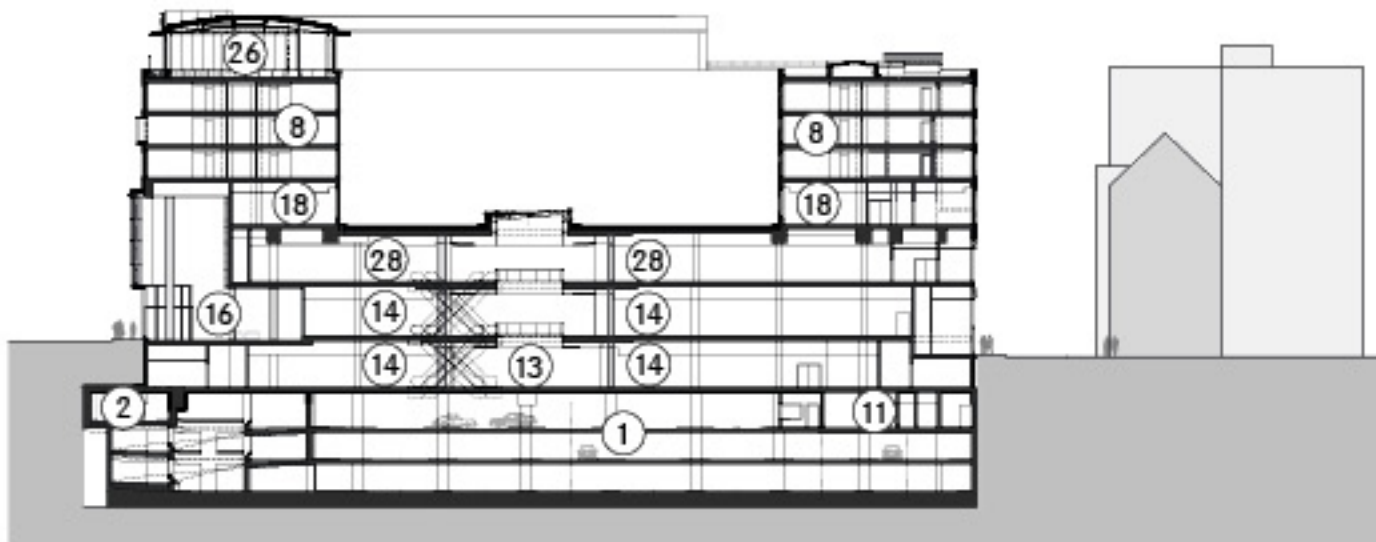
Schnitt Q7
