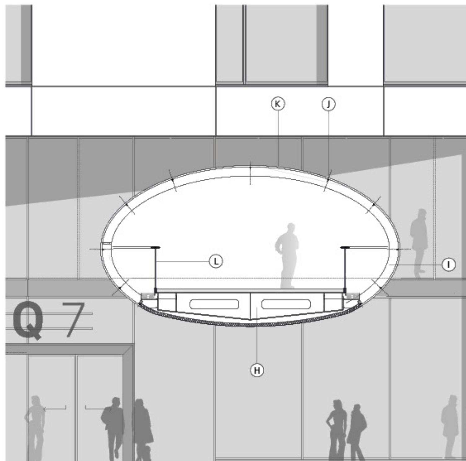
Querschnitt Brücke
