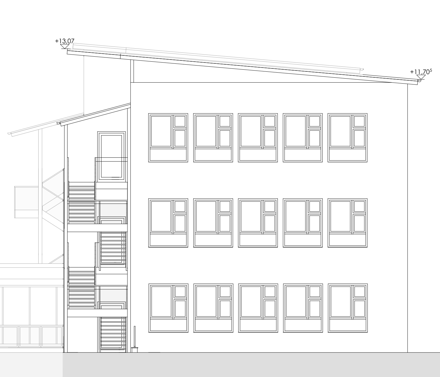
WESTANSICHT
