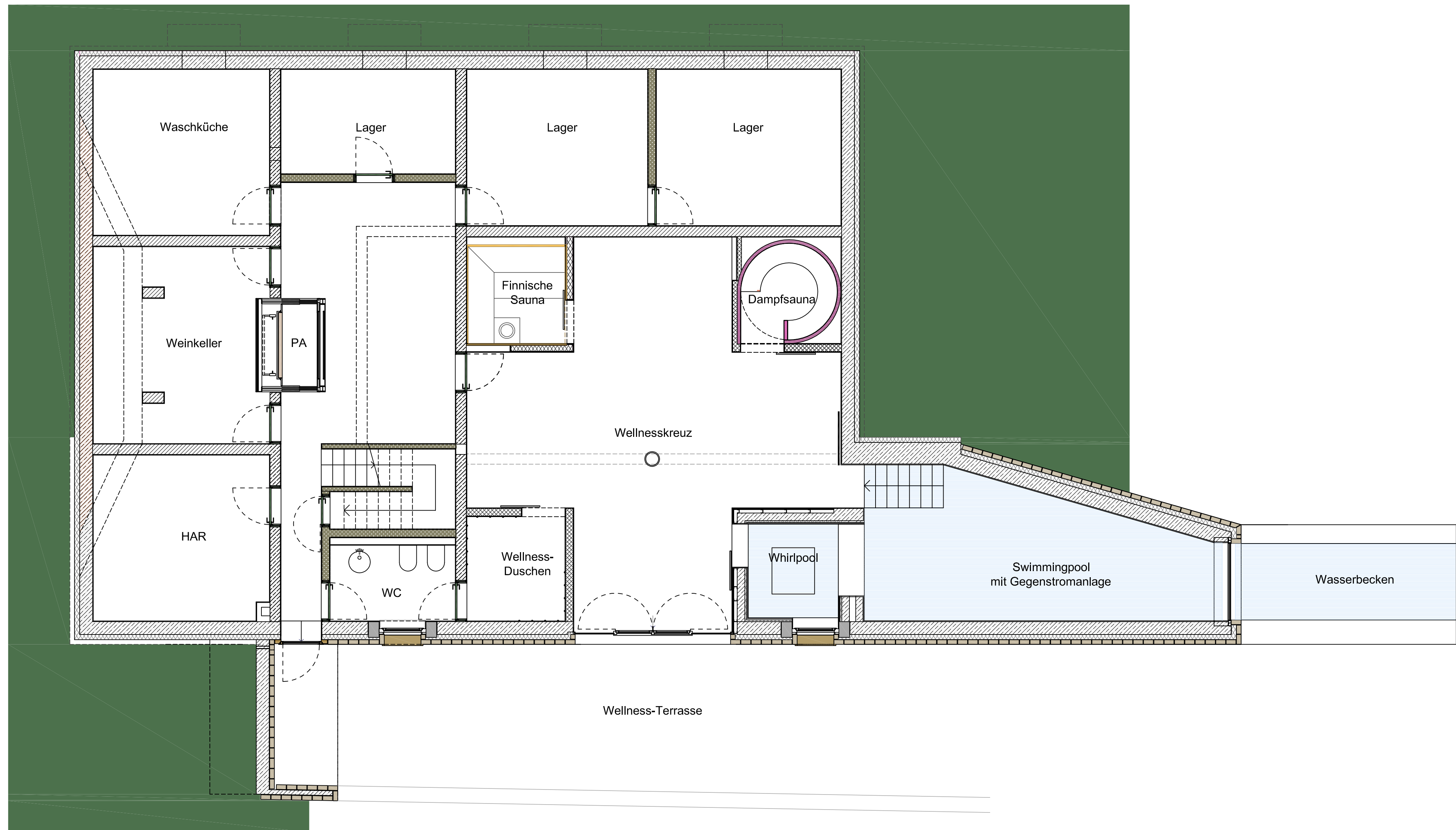
Gartengeschoss
