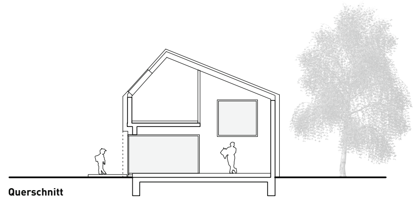
Querschnitt
