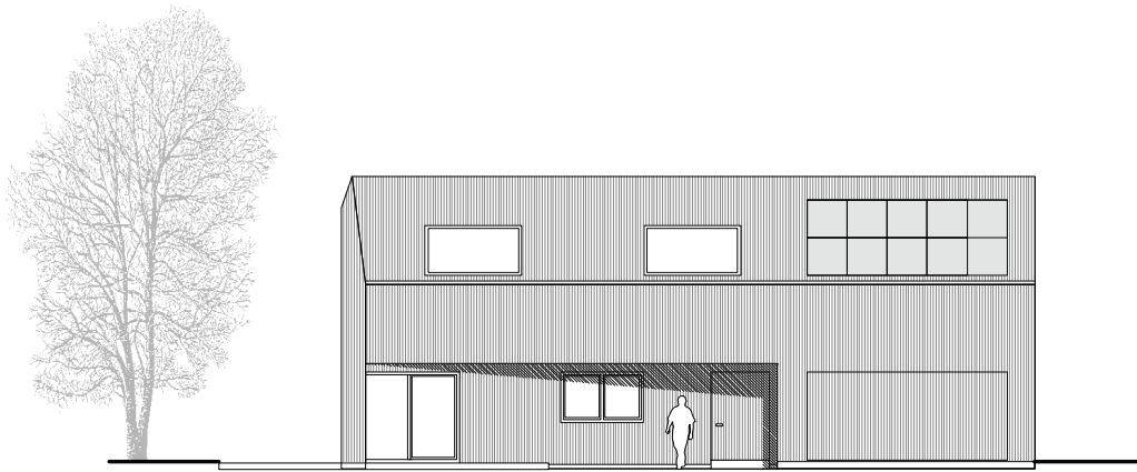
Ansicht Süd
