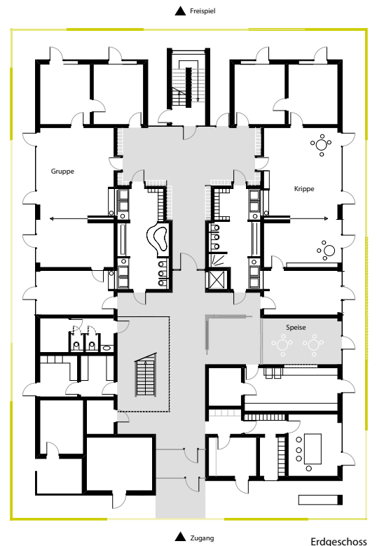
Erdgeschoss
