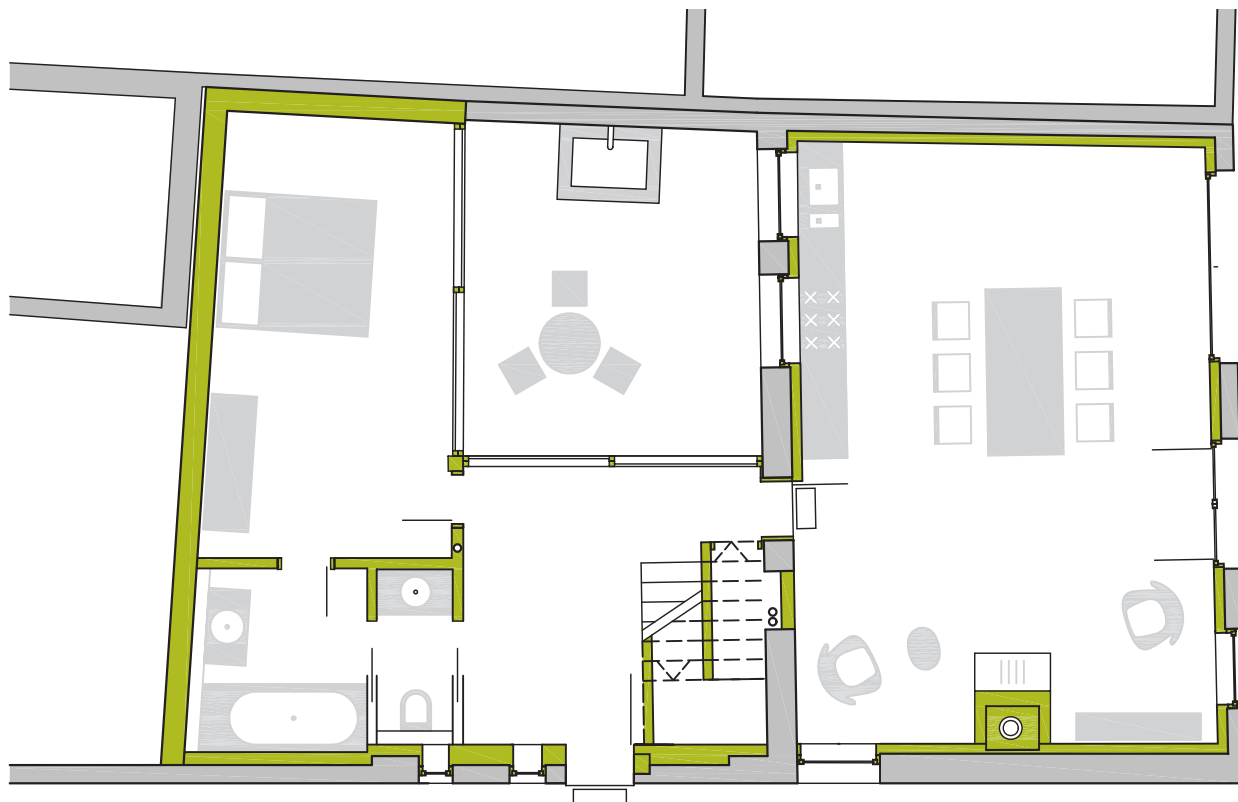
EG M 1-100
