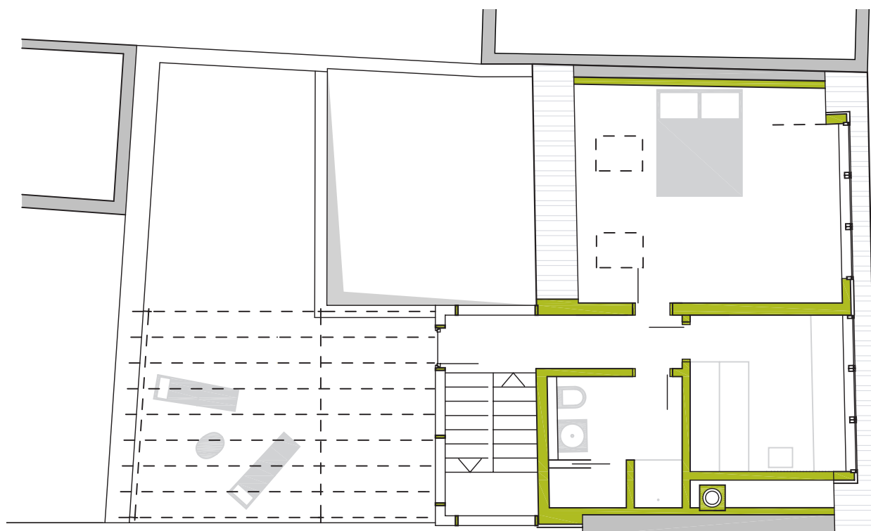
OG M 1-100
