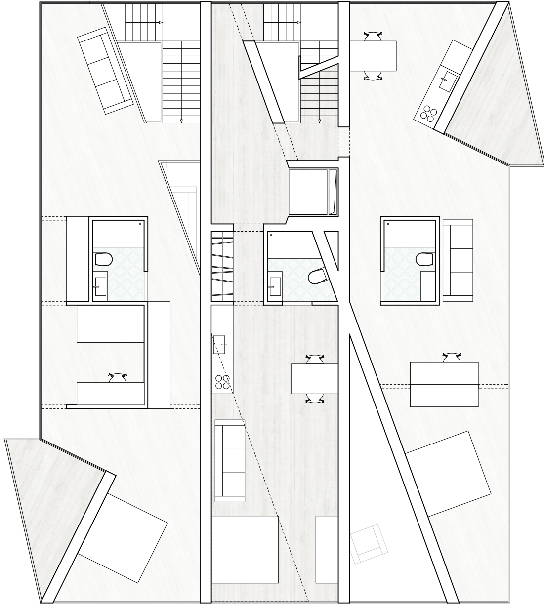
5. OG M 1:100
