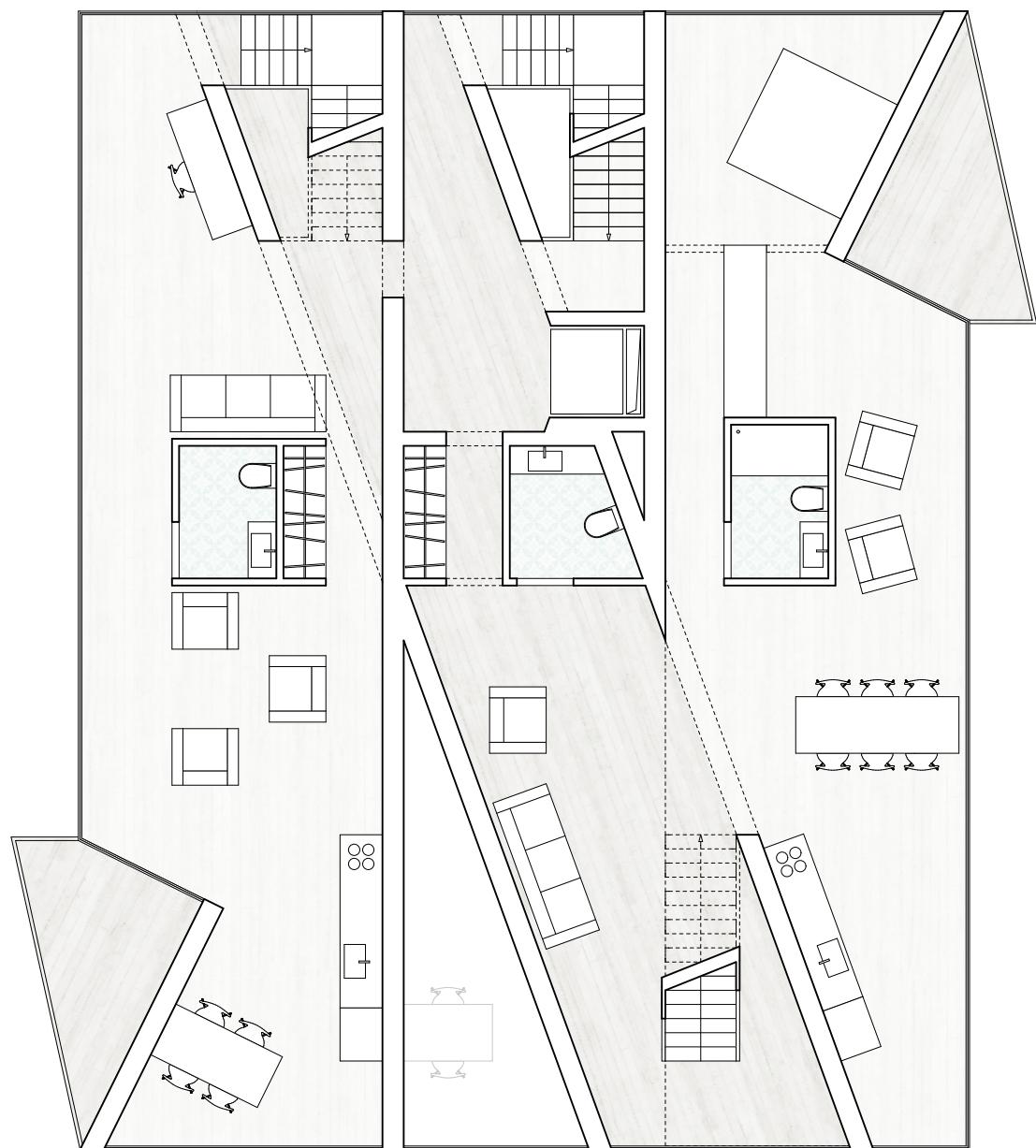
2. OG M 1:100
