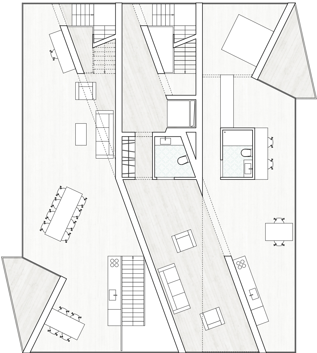
4. OG M 1:100
