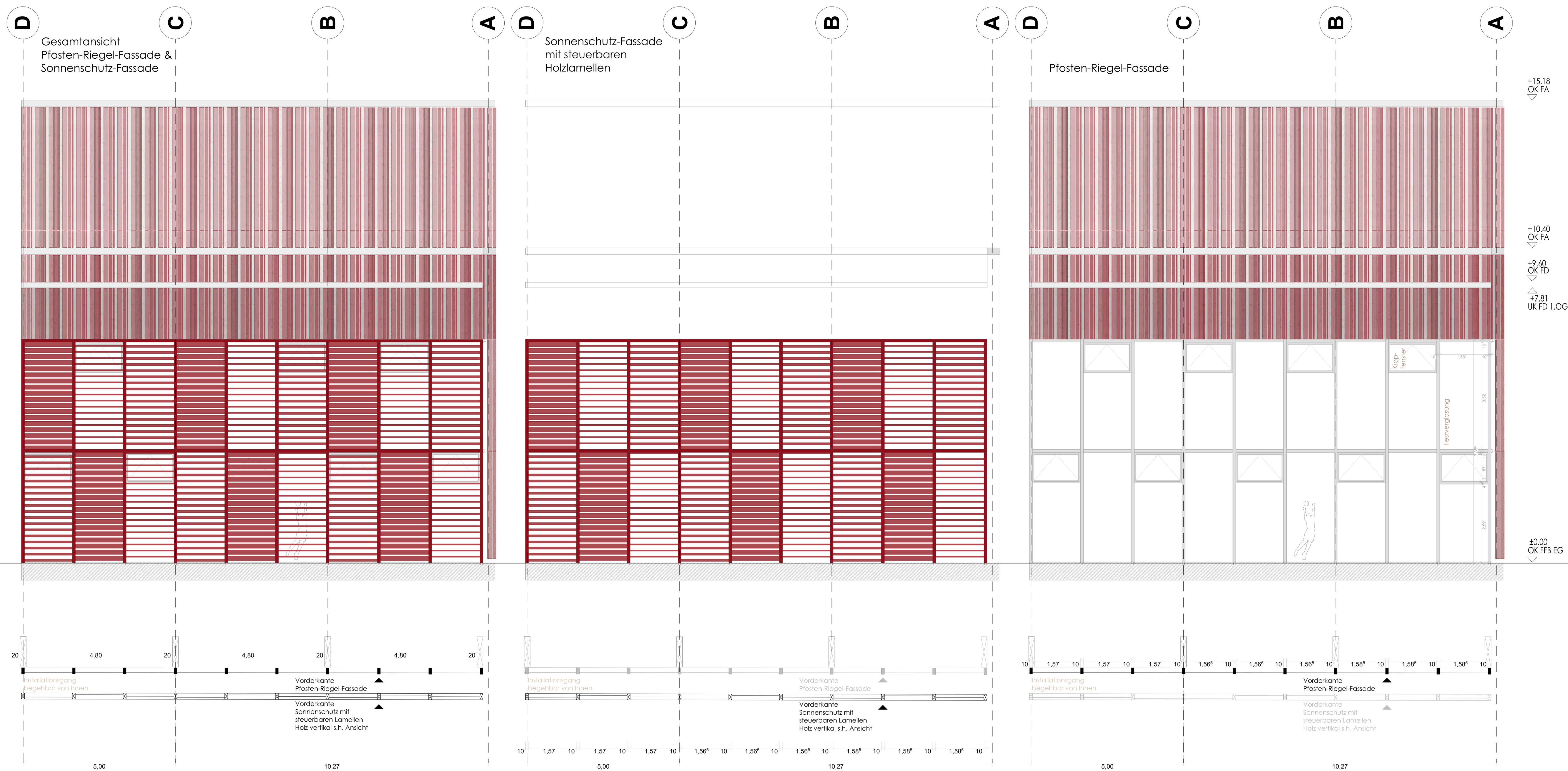
Darstellung der verschiedenen Schichten Fassadenansicht Süd-West Sporthalle 1:50
