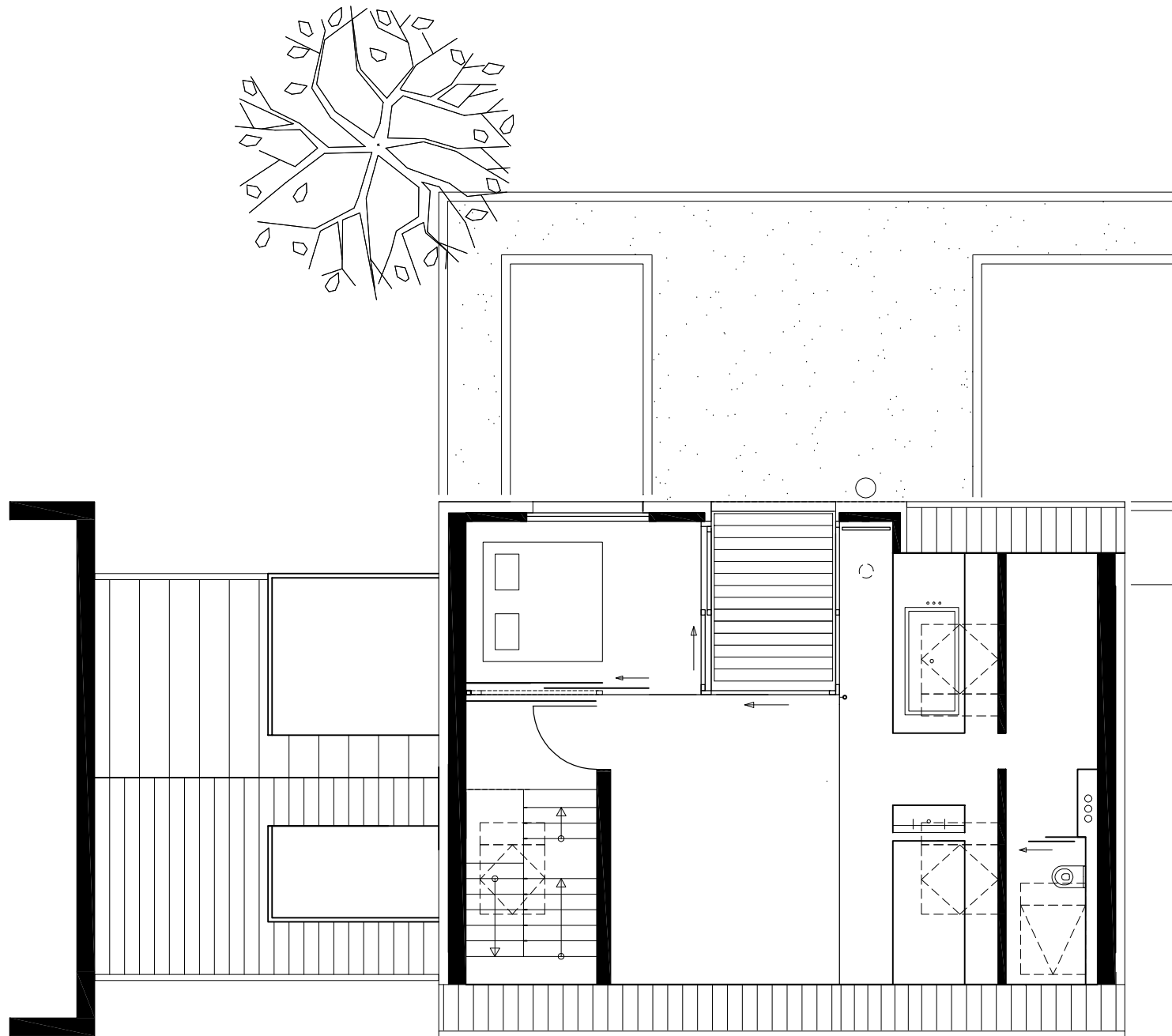
⊕ Dachgeschoss M1:100
