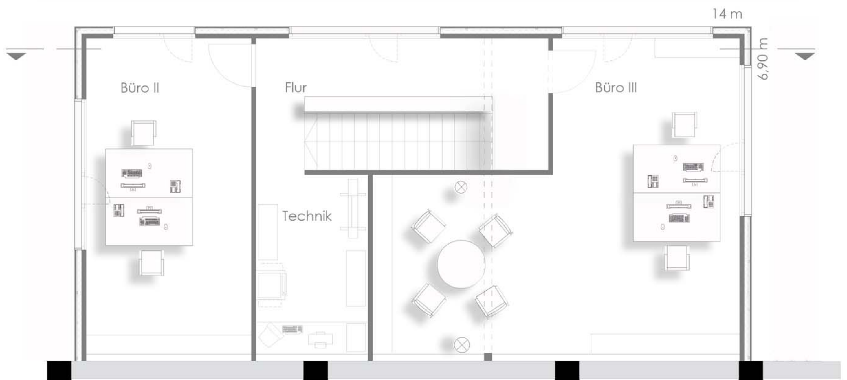
Grundriss Büro Obergeschoss
