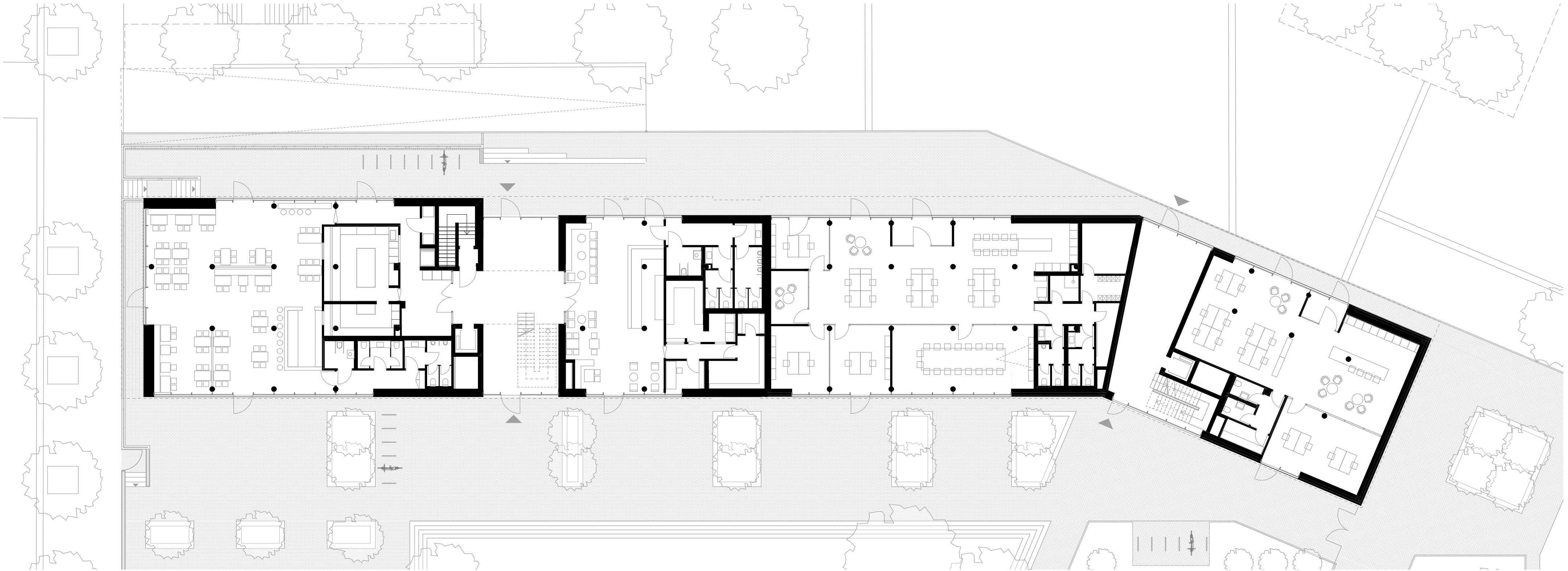
GRUNDRISS EG | M 1.200
