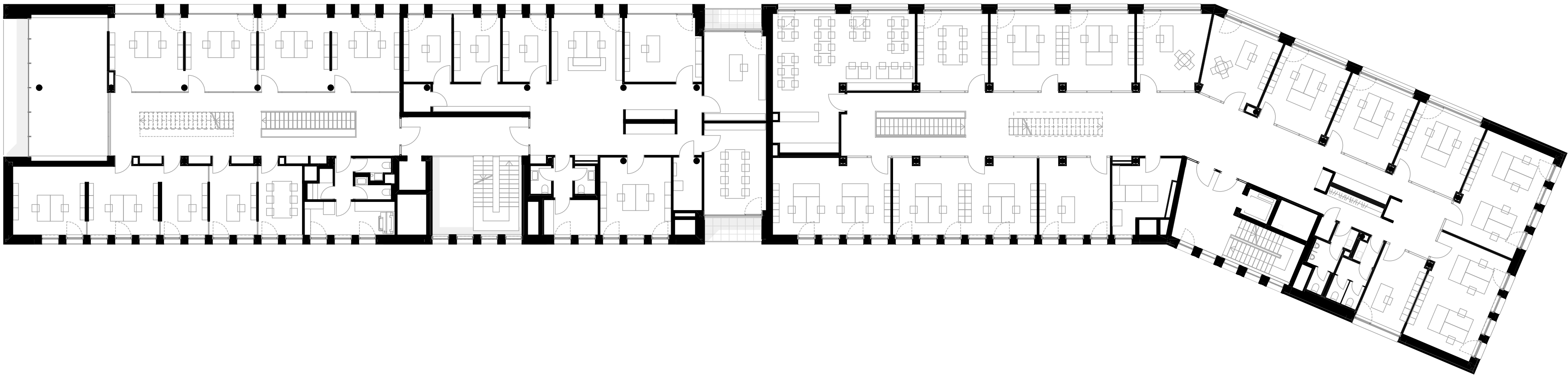
GRUNDRISS 2.OG | M_1.200
