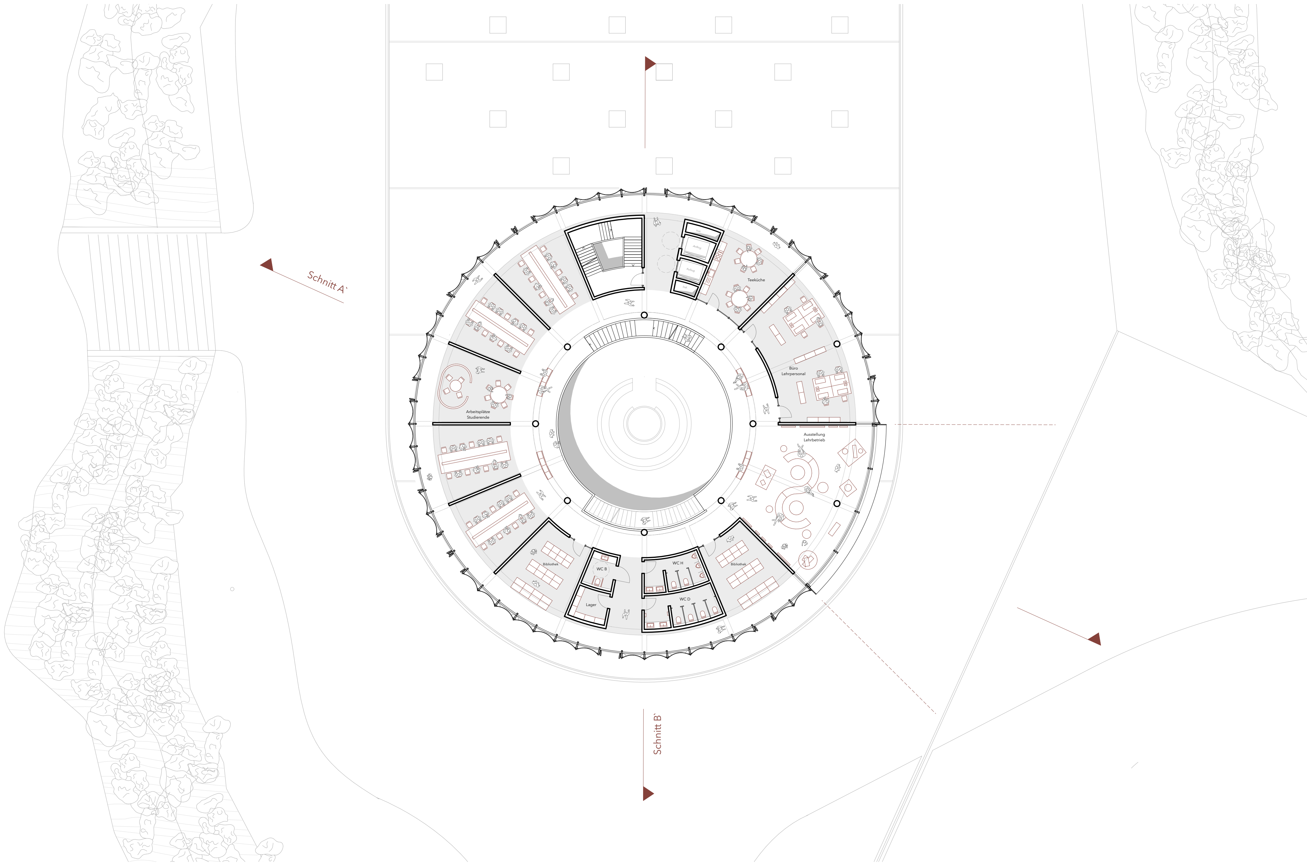
Grundriss 2. Obergeschoss M 1 : 200
