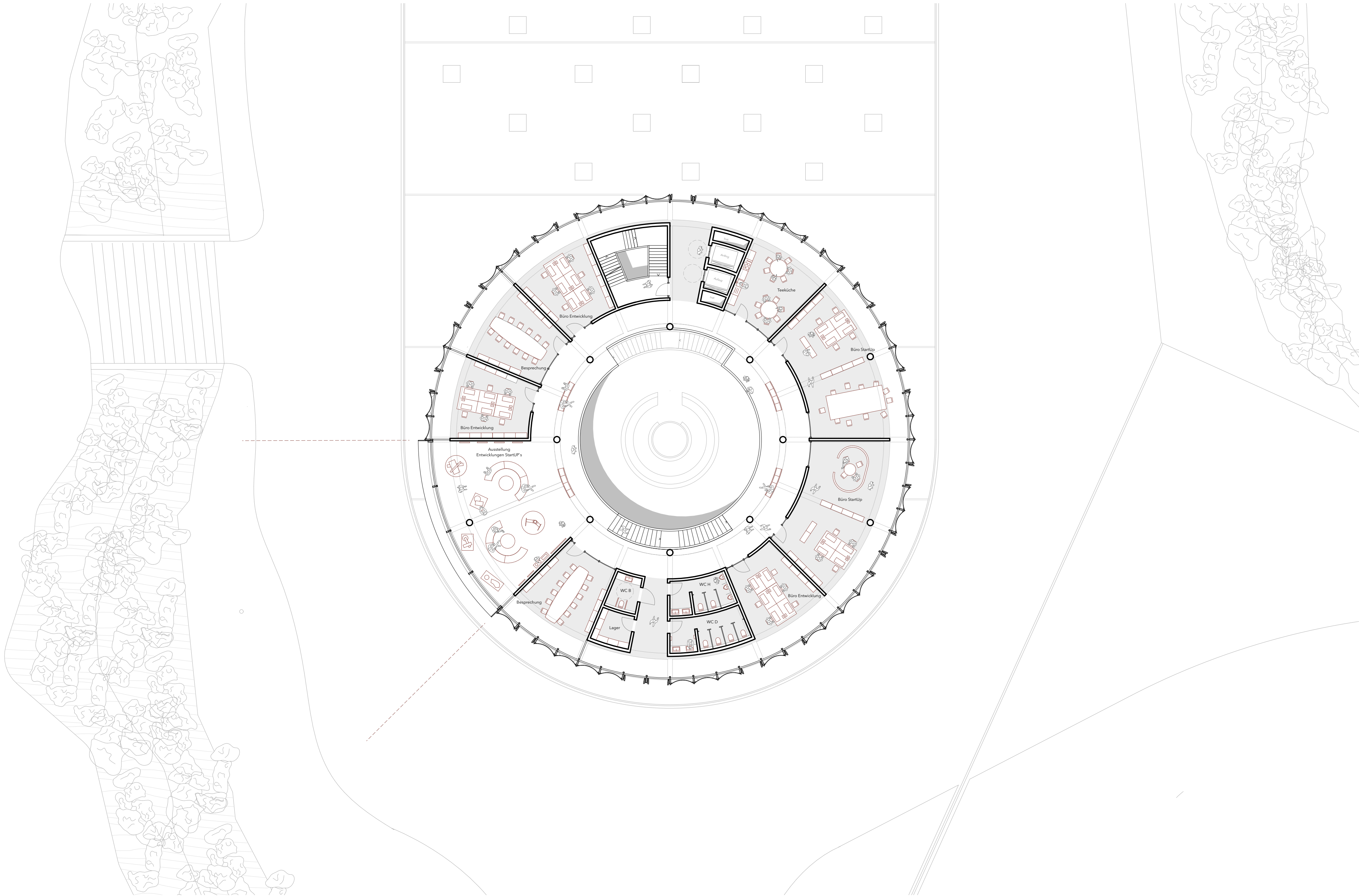
Grundriss 3. Obergeschoss M 1 : 200
