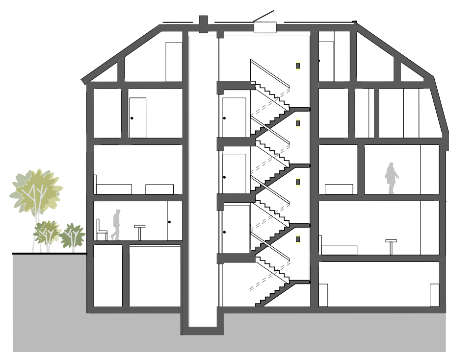
Schnitt A-A M1:200
