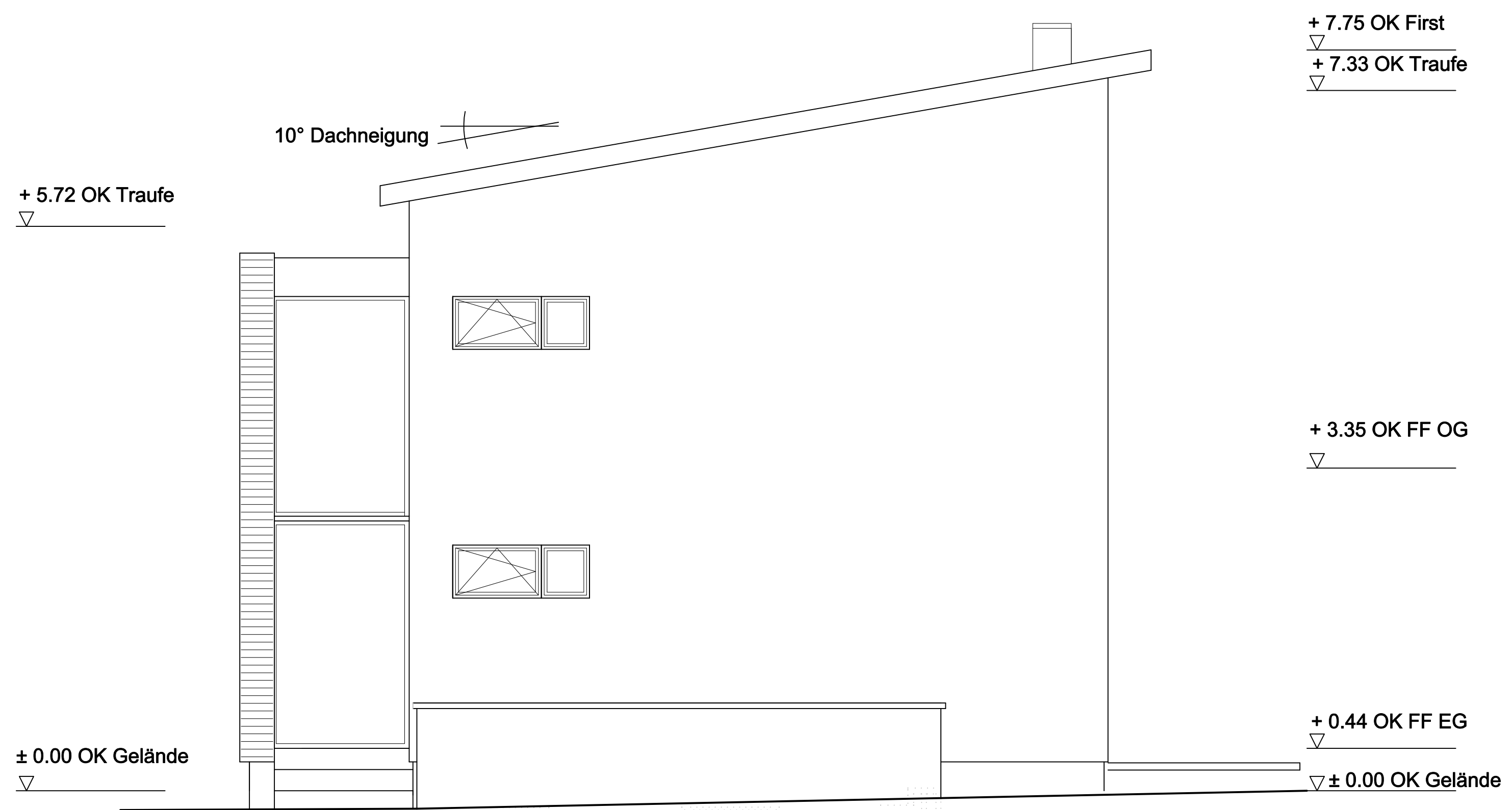
Nord Ansicht
