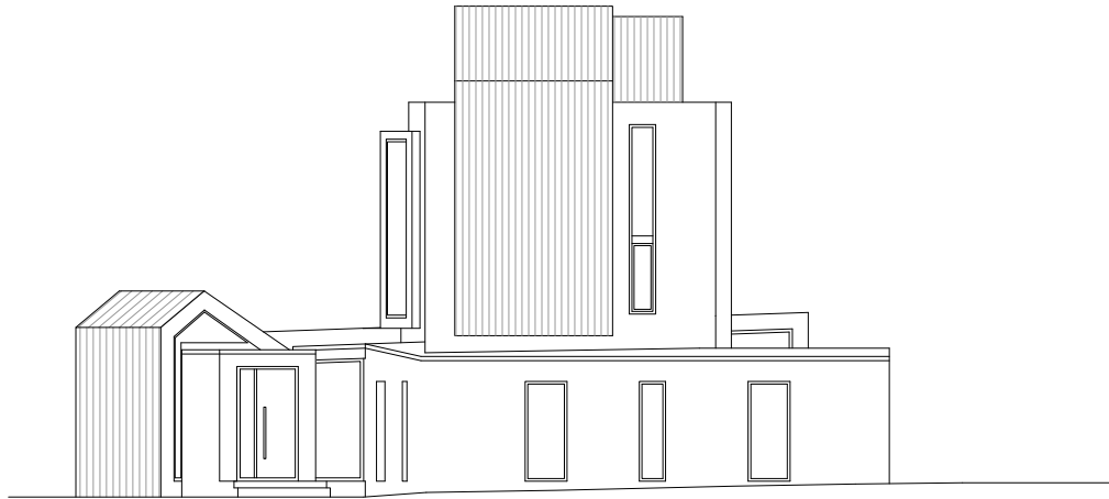
Ansicht Süd-West
