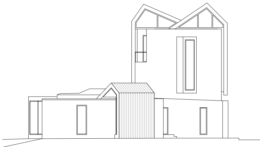
Ansicht Nord-West
