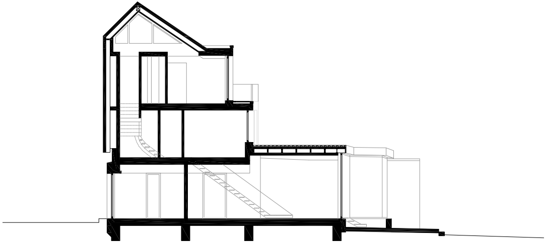
Schnitt A-A
