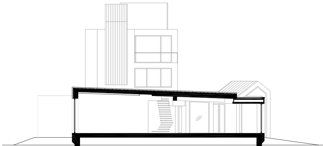
Schnitt B-B
