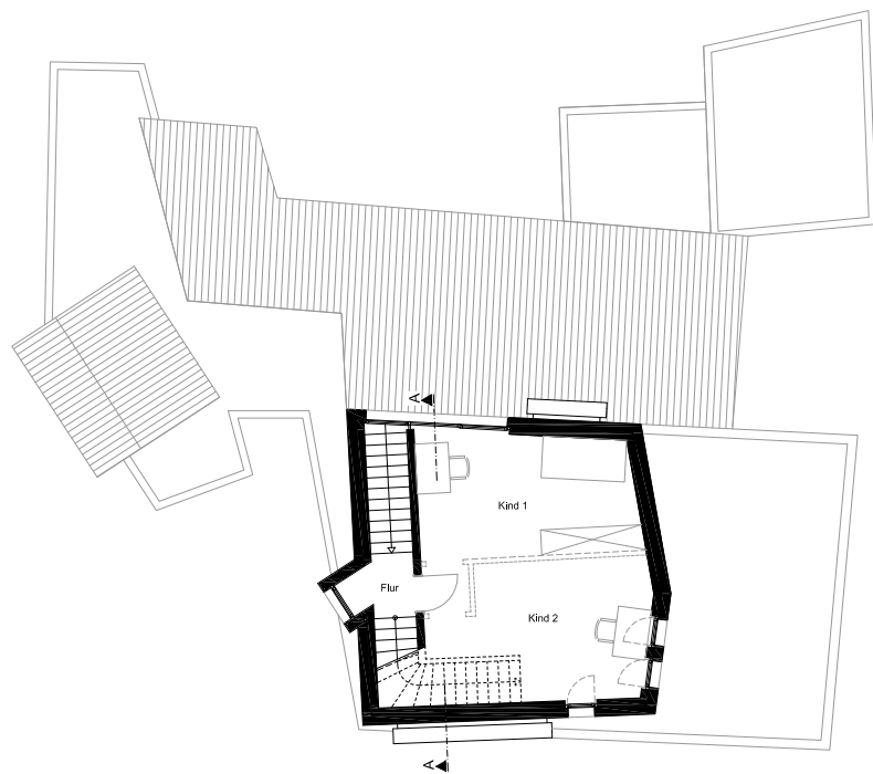
Grundriss 1. Obergeschoss
